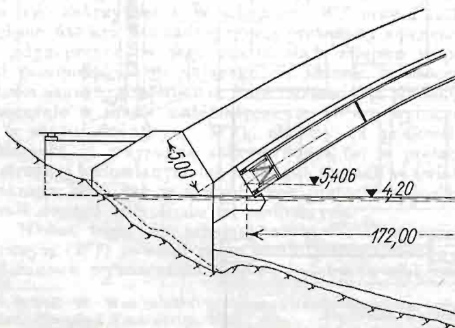
Rys. 6. Oparcie węzłowania rusztowania łuku.
