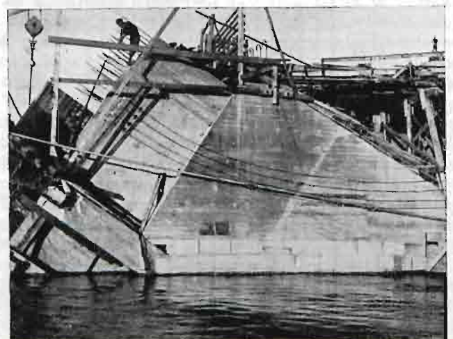
Ryc. 7. Węzłowie łuku.
