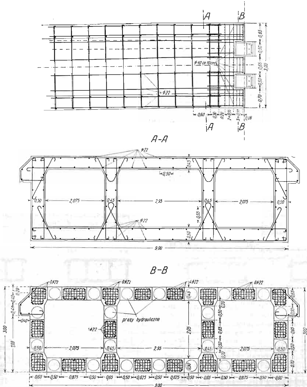
Rys. 5. Szczyt klucza łuku z przekrojami.
