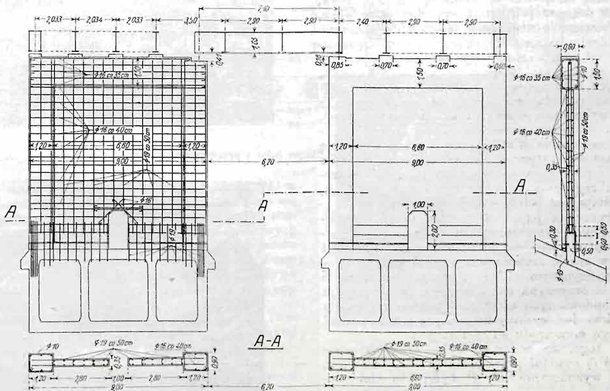
Rys. 4. Ustrój jednego z filarów ściennych.
