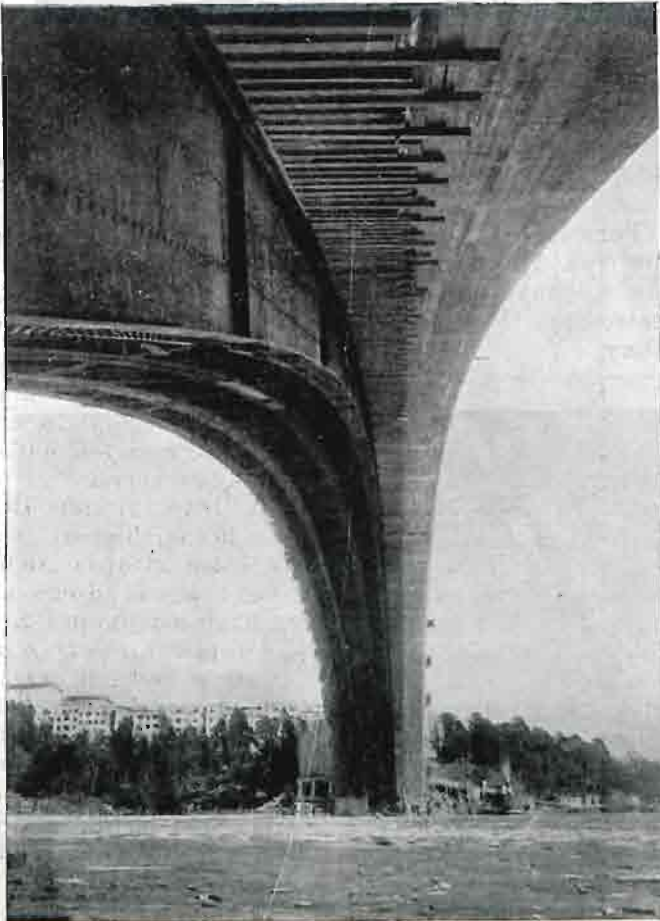
Ryc. 13. Spód łuku w okresie przesuwania rusztowania stalowego.
