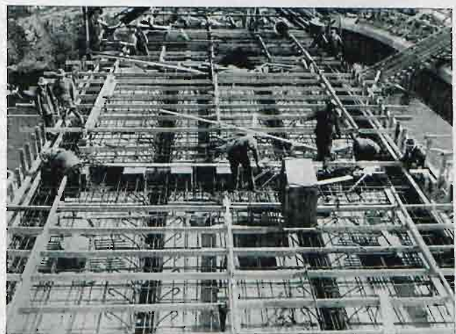
Ryc. 11. Fragment układania wkładek łuku.
