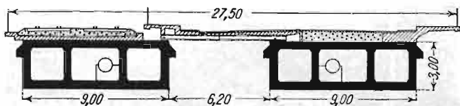
Rys. 2. Przekrój łuku w kluczu.
