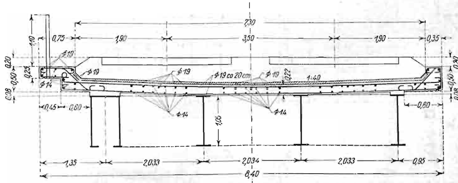
Rys. 1. Normalny przekrój pomostu.
