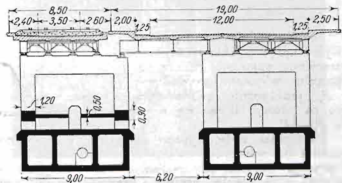
Rys. 3. Przekrój łuku w 1/4.
