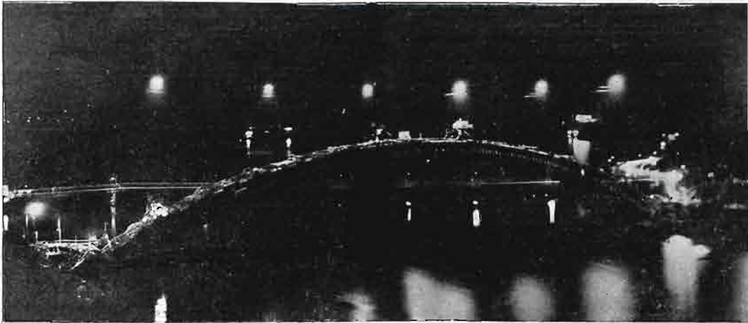
Ryc. 15. Fragment wykonania łuku przy sztucznym oświetleniu. W głębi dotychczasowy most pływający (pontonowy).
