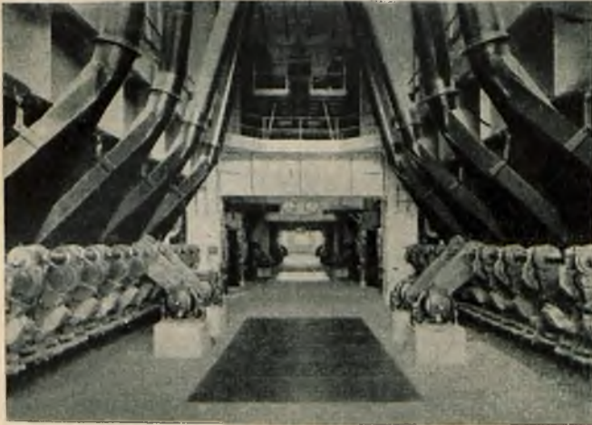
Rys. 12. Kociołnia elektrowni West.
