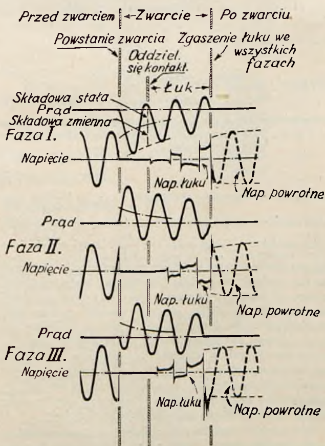
Rys. 5. Typowe oscylogramy zwarcia trójfazowego.
