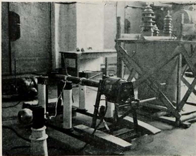
Rys. 5. Prostownik mechaniczny z laboratorium „Ćmielowa”
