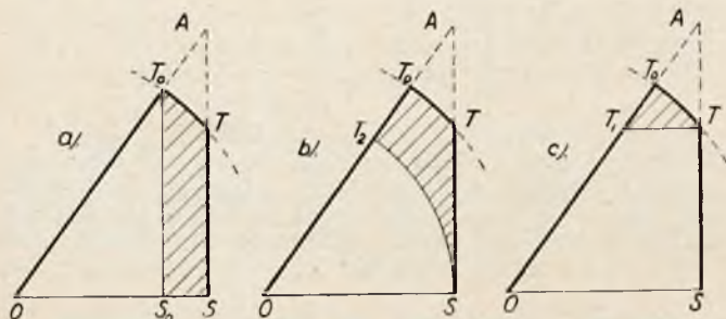
Rys. 4. Wykresy, odpowiadające rys. 3, na których zaznaczony jest zakres (pola zakreślane), w których wyłącznik działa prawidłowo, a który wykluczają od stosowania projekty 1, 2 i 3 (odpowiednie wykresy a, b i c).
