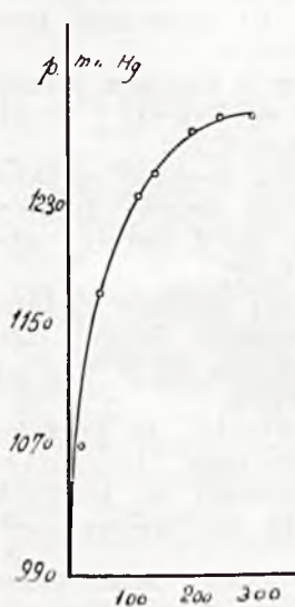
Rycina 9. Przyrost ciśnienia gazu p z postępowaniem reakcji w doświad. Nr 61.
