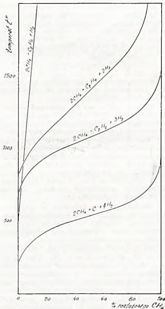
Rycina 1. Zależność stopnia dysocjacji metanu od temperatury.
