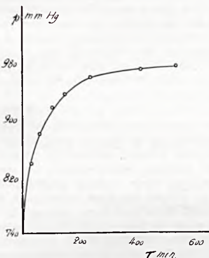
Rycina 9. Przyrost ciśnienia gazu p z postępowaniem reakcji w doświad. Nr 61.
