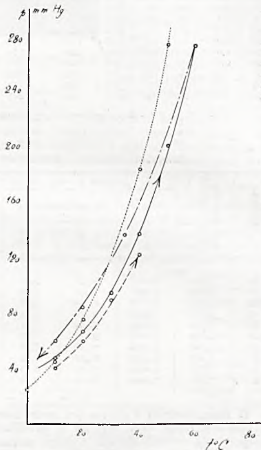
Rycina 7. Krzywe prężności par nasyconych p kondensatu z doświadczeń Nr 51.
