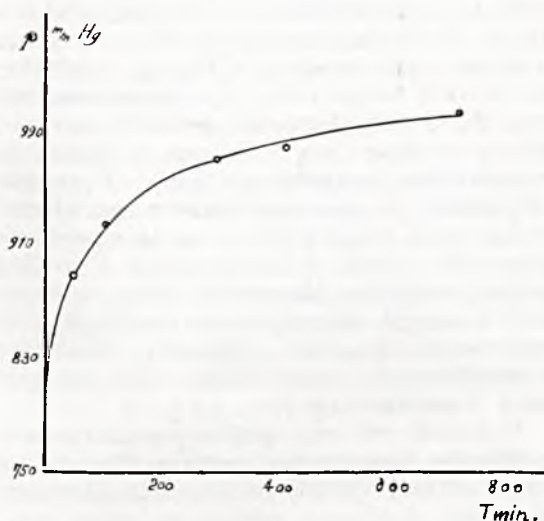
Rycina 8. Przyrost ciśnienia gazu p z postępowaniem reakcji w doświad. Nr 51.
