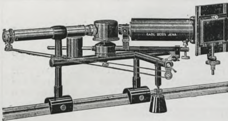
Uniwersalny spektrograf Zeiss'a Model II, z kasetą 9×12 cm
