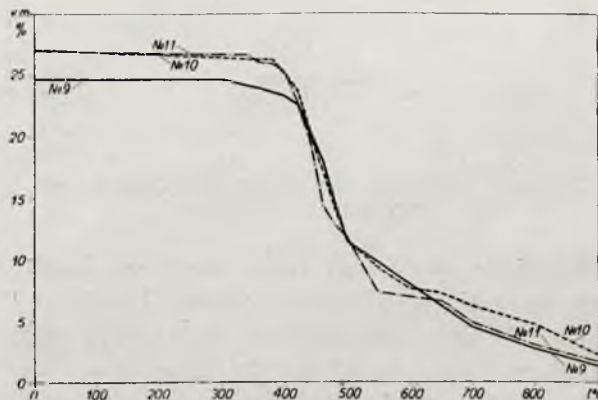
Rycina 2. Przebieg odgazowania typowych węgla koksowniczych.
