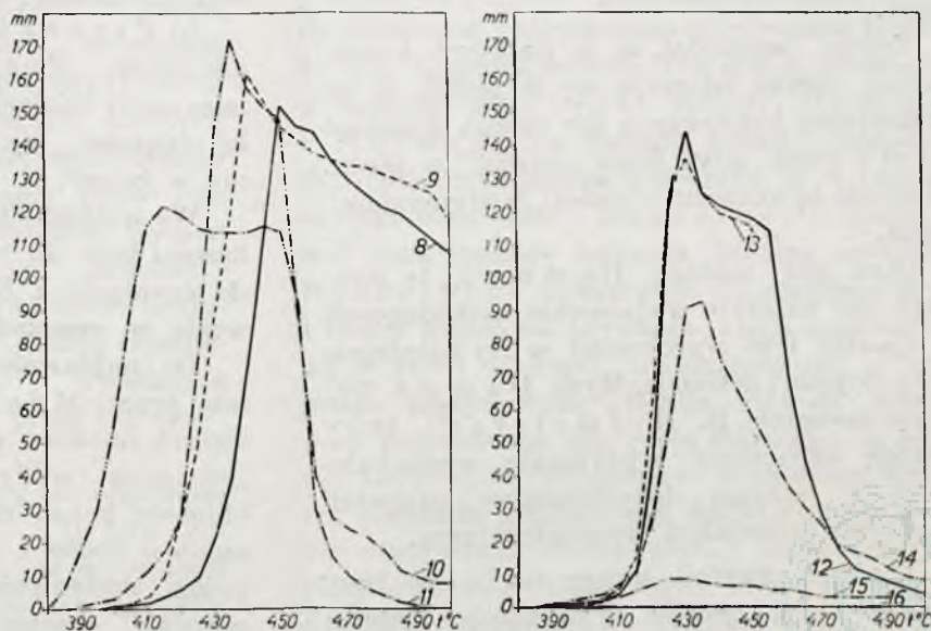
Rysunek 6. Krzywe plastyczności: a) węgli koksowniczych, b) węgli gazowych.
