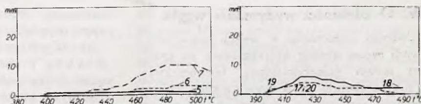
Rysunek 5. Krzywe plastyczności: a) węgli chudych, b) węgli gazowopłomiennych.
