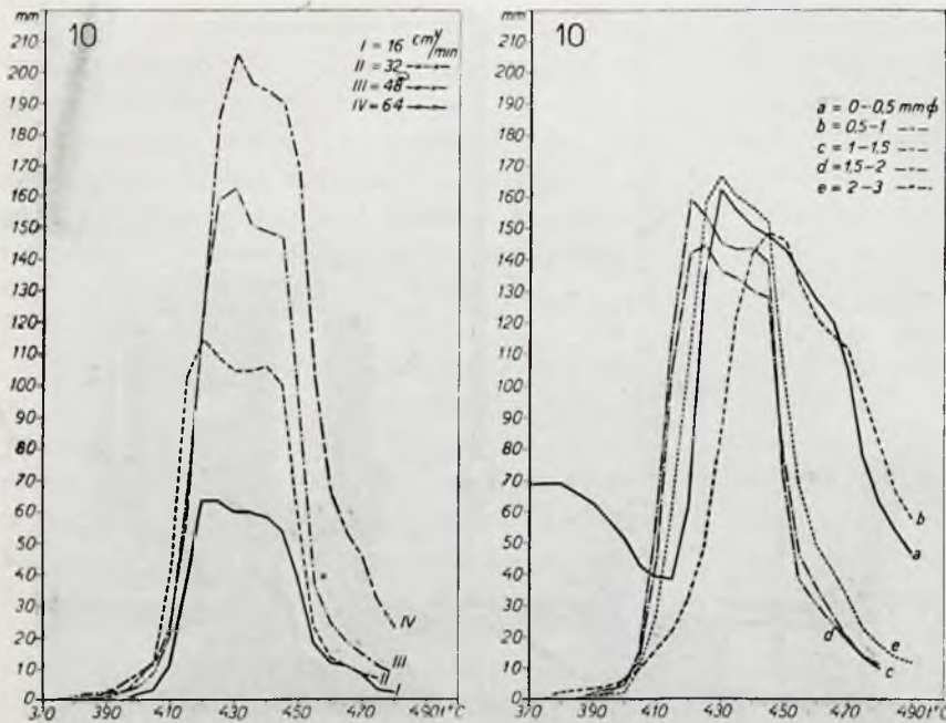
Rysunek 3. Krzywe plastyczności węgla.
