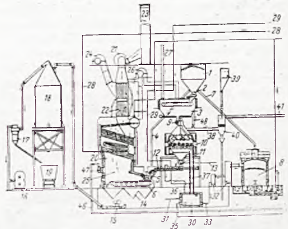
Załączony rysunek przedstawia schematycznie instalację Merz'a i Mc. Lellana .
