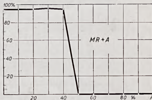
Rys. 13. Wytrzymałość na ścieranie brykietów z mieszaniny węgla koksującego z niekoksującym (zmienny skład procentowy mieszaniny).
