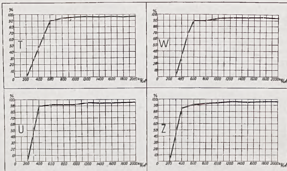
Rys. 12. Wytrzymałość na ścieranie brykietów z górnośląskich węgli niekoksujących (zmiennie ciśnienie).
