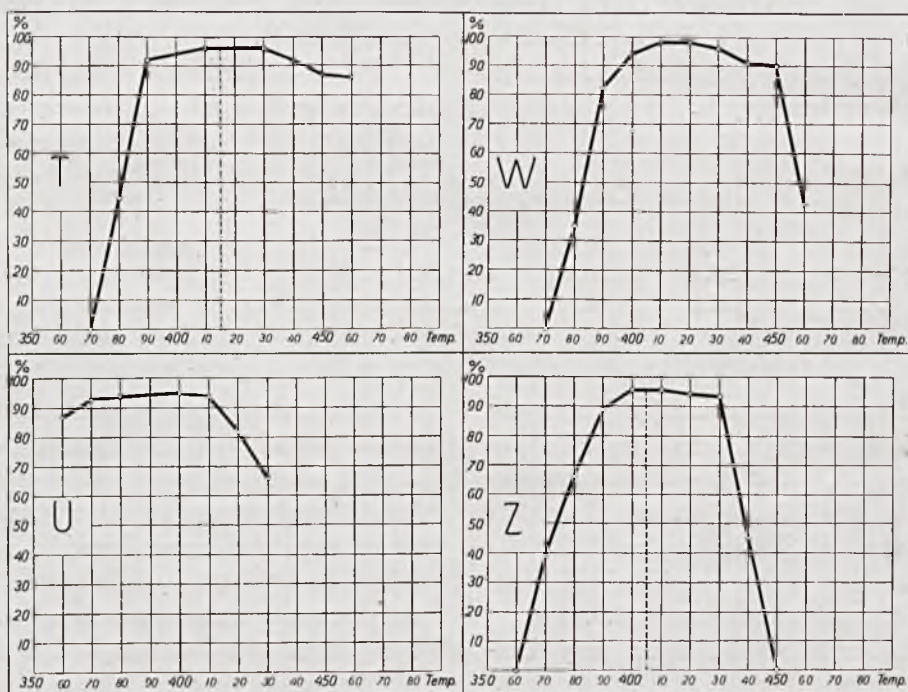
Rys. 8. Wytrzymałość na ścieranie brykietów z górnośląskich węgli niekoksujących (zmienna temperatura).
