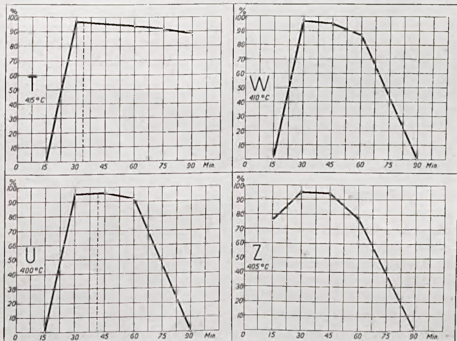
Rys. 11. Wytrzymałość na ścieranie brykietów z górnośląskich węgli niekoksujących (zmienny czas ogrzewania).
