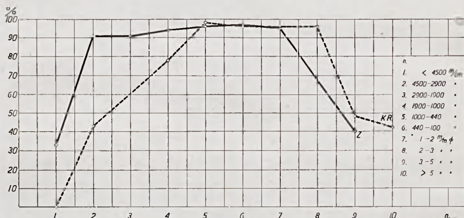
Rys. 18. Wytrzymałość na ścieranie brykietów z węgla niekoksujących (zmienna wielkość ziarna).
