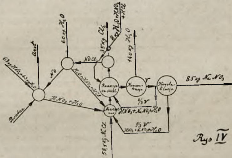
Schemat fabrykacji saletry i chloru z chlorków i 50%-owego \text{HNO}_3 .
