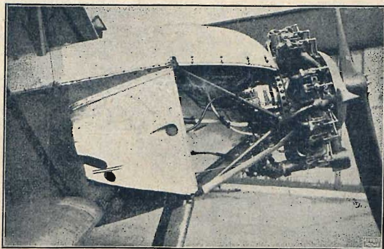
BARTEL BM 2. Motyw przedniej części kadłuba wykazujący umocowanie silnika. Zauważyć należy wielką łatwość dostępu do każdej części.
