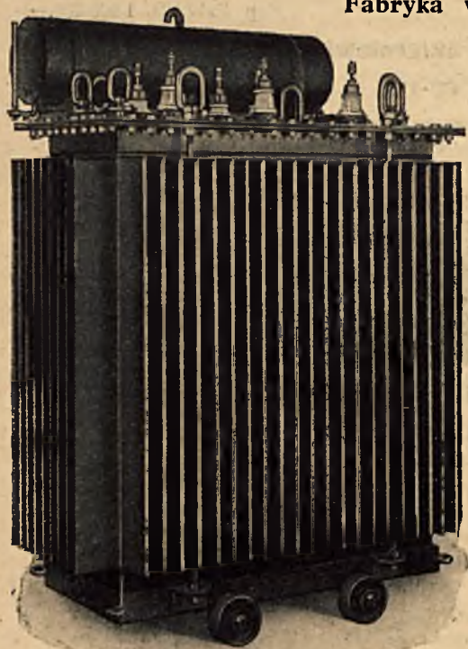
Transformator 3-fazowy 800 kVA
