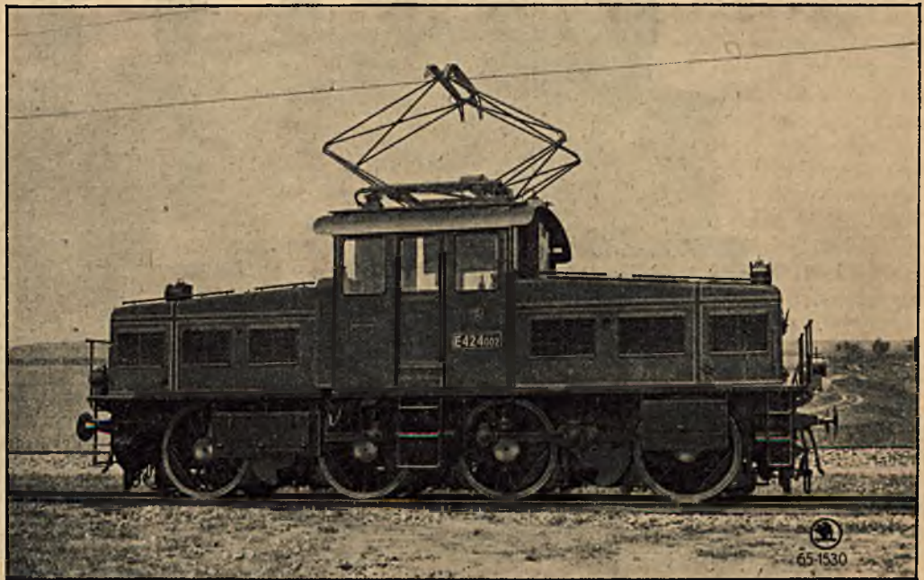
Elektryczna lokomotywa do pociągów towarowych typ B—B na prąd stały 1 500 V o wadze 58 ton
