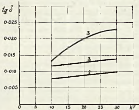
Rys. 5. Zmiany kąta stratności w funkcji napięcia pod wpływem ogrzania.
