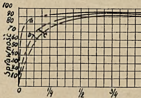
Rys. 7. Obciążenie.
