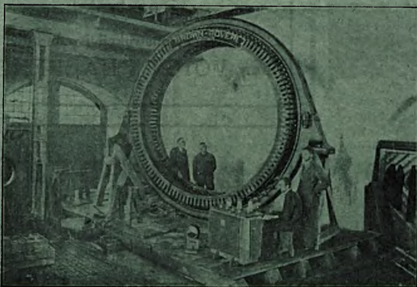
Prądnica trójfazowa o mocy 780 kVA, 550 V, 187 obr. min. wykonywana w fabryce w Żychlinie dla Elektrowni Miejskiej w Tarnowie.
