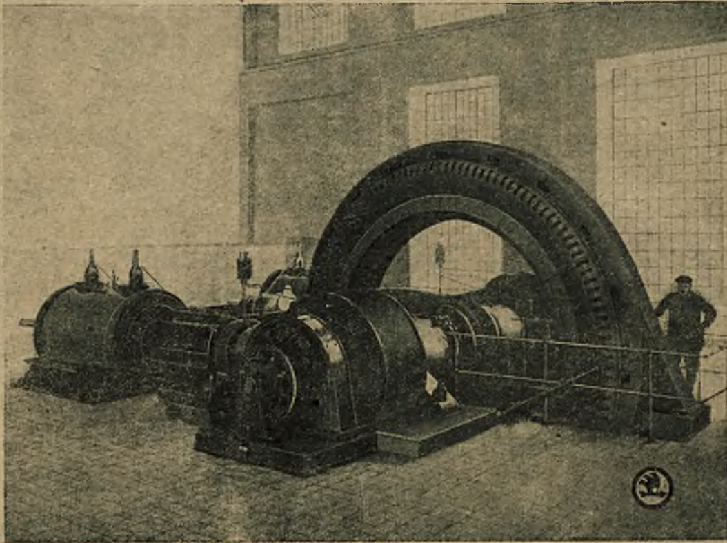
Generator prądu trójfazowego 2000 KVA, 115 obrotów. 400/231 volt. Cukrownia Hodonin.
