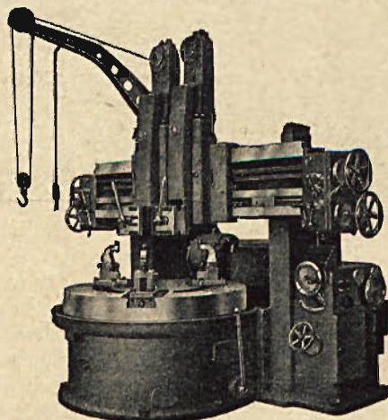
»Tokarka karuzelowa do obręczy i kół typ 1 KBE«
