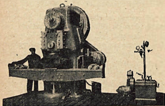
»Prasa do statycznego i dynamicznego próbowania resorów typ PS«
