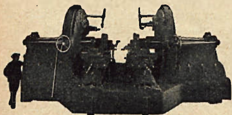
»Tokarka do zestawów kołowych typ 3 TC«
