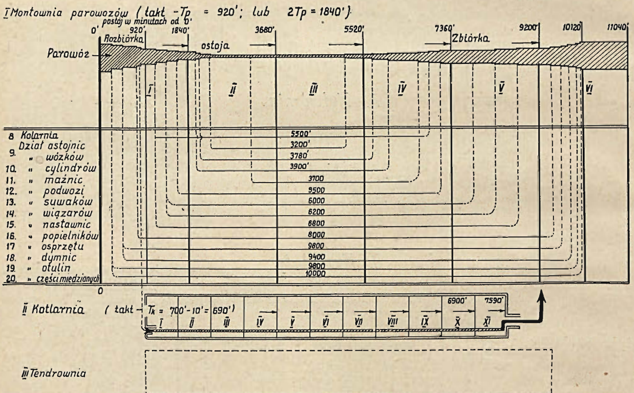
Rys. 6. Orientacyjny harmonogram robót w naprawniach.
