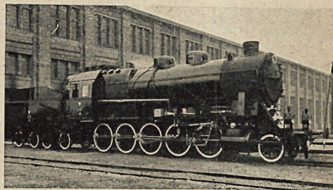
Rys. 2. Parowóz serii Ty 23 (1—5—0) zbudowany w wytwórni H. Cegielski.
