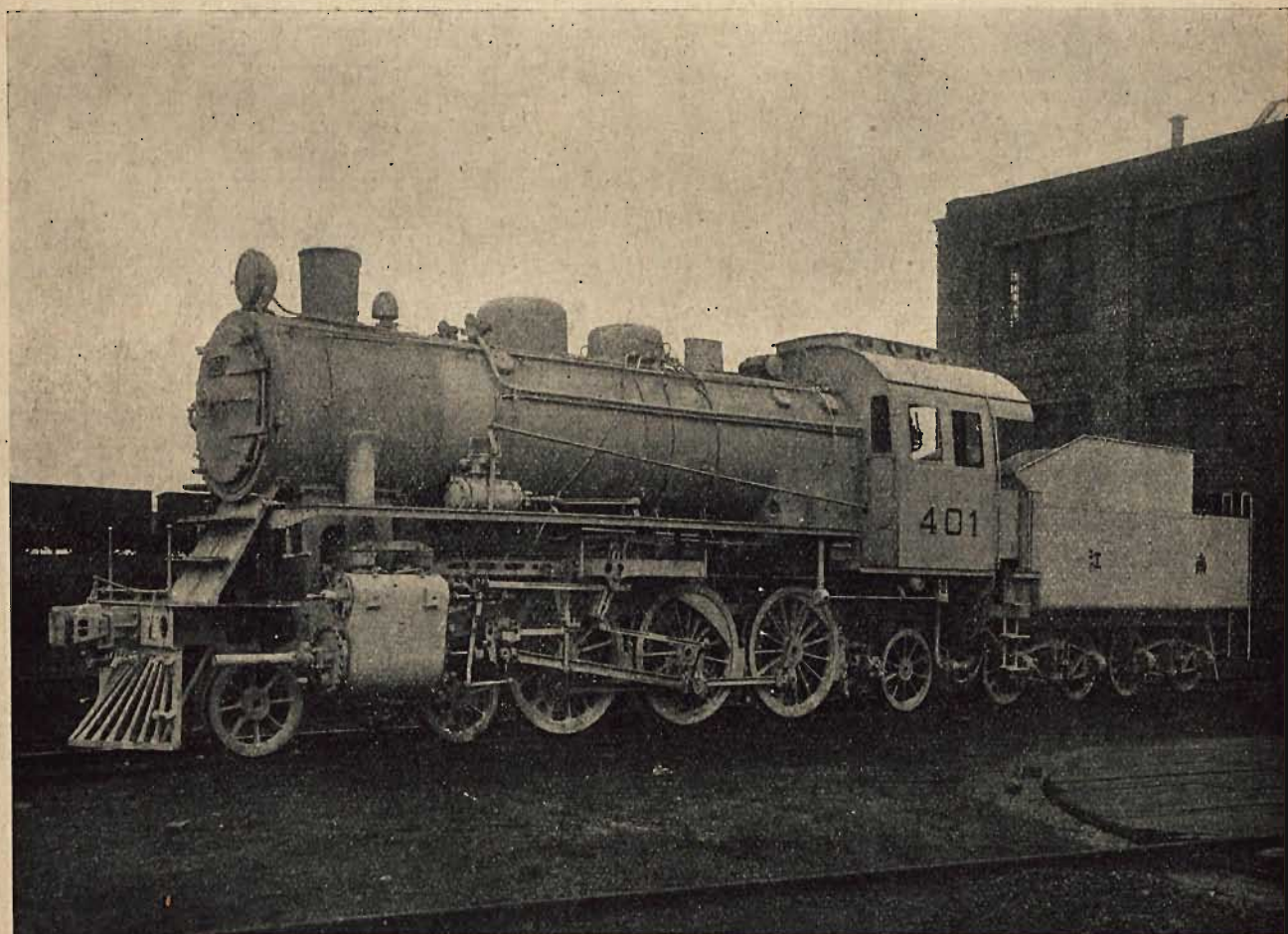
Parowóz do pociągów pociągów typu Pacific, zbudowany w zakładach Sp. Akc. H. Cegielski w Poznaniu dla kolei chińskich Kjangnan.
