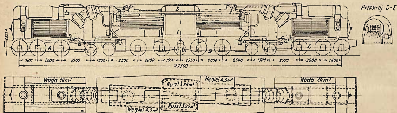
Parowóz trójczłonowy typu „Franco”
