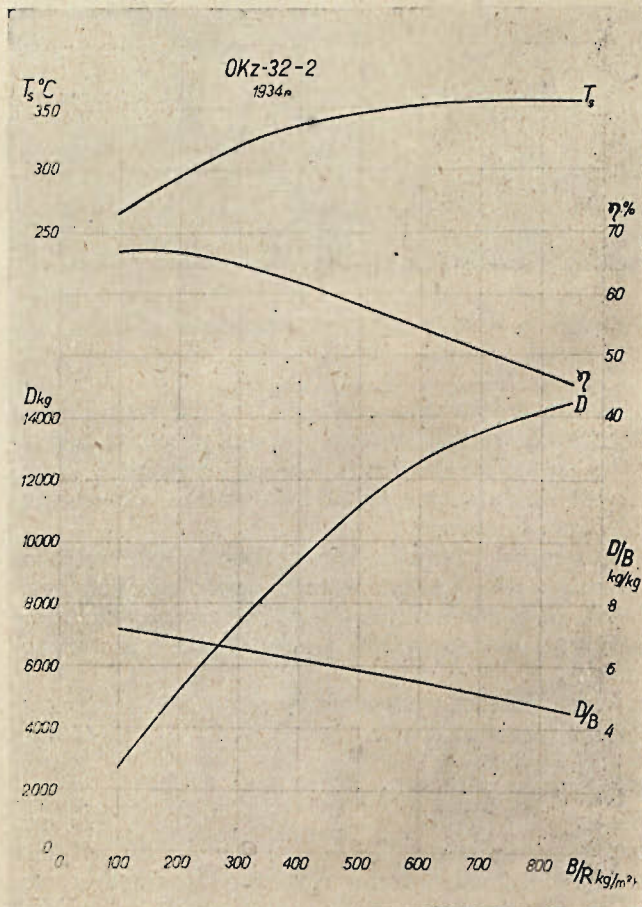
Rys. 9. Krzywe kotłowe w zależności od natężenia rusztu.
