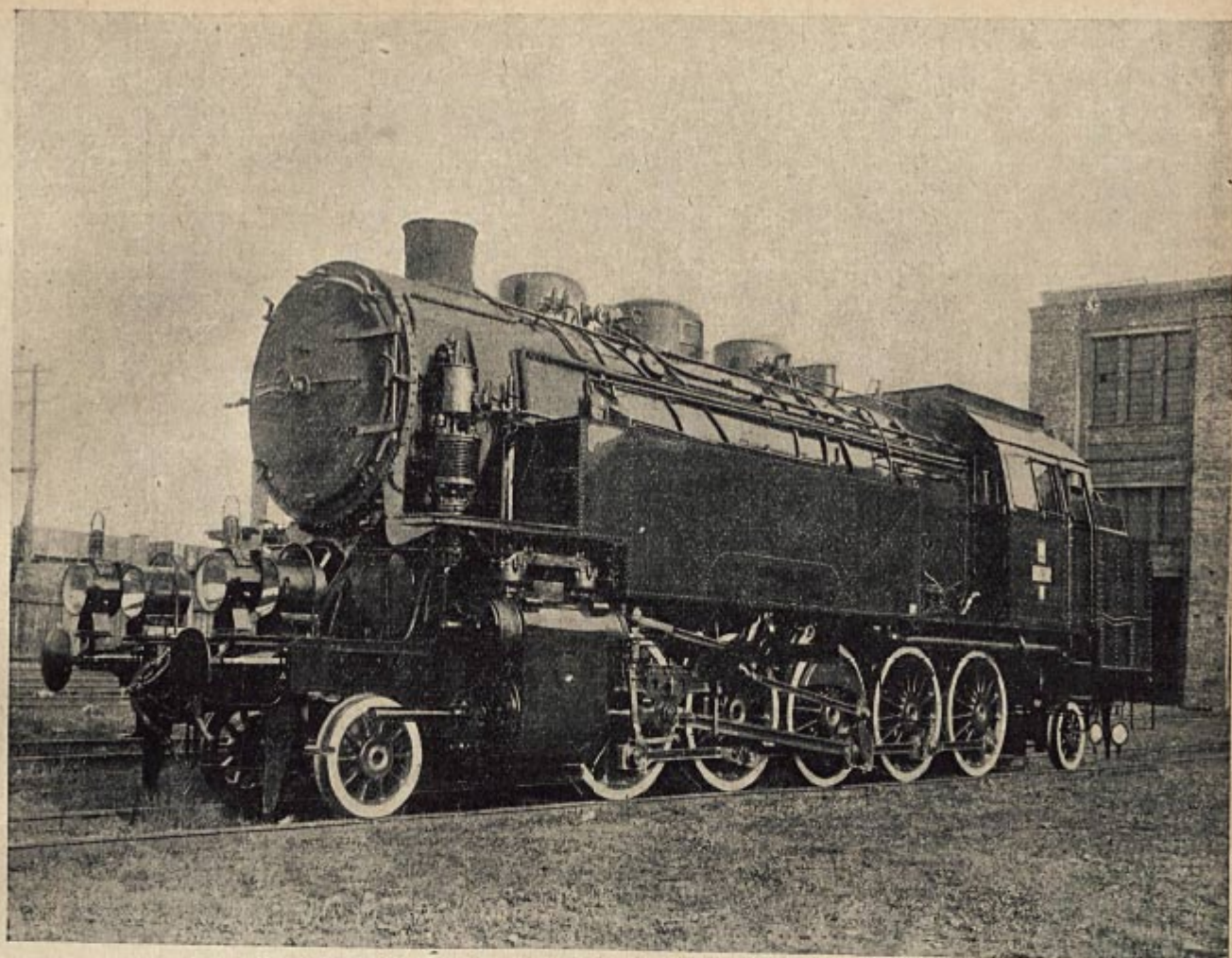
Rys 1. Widok ogólny parowozu serii OKz32.
