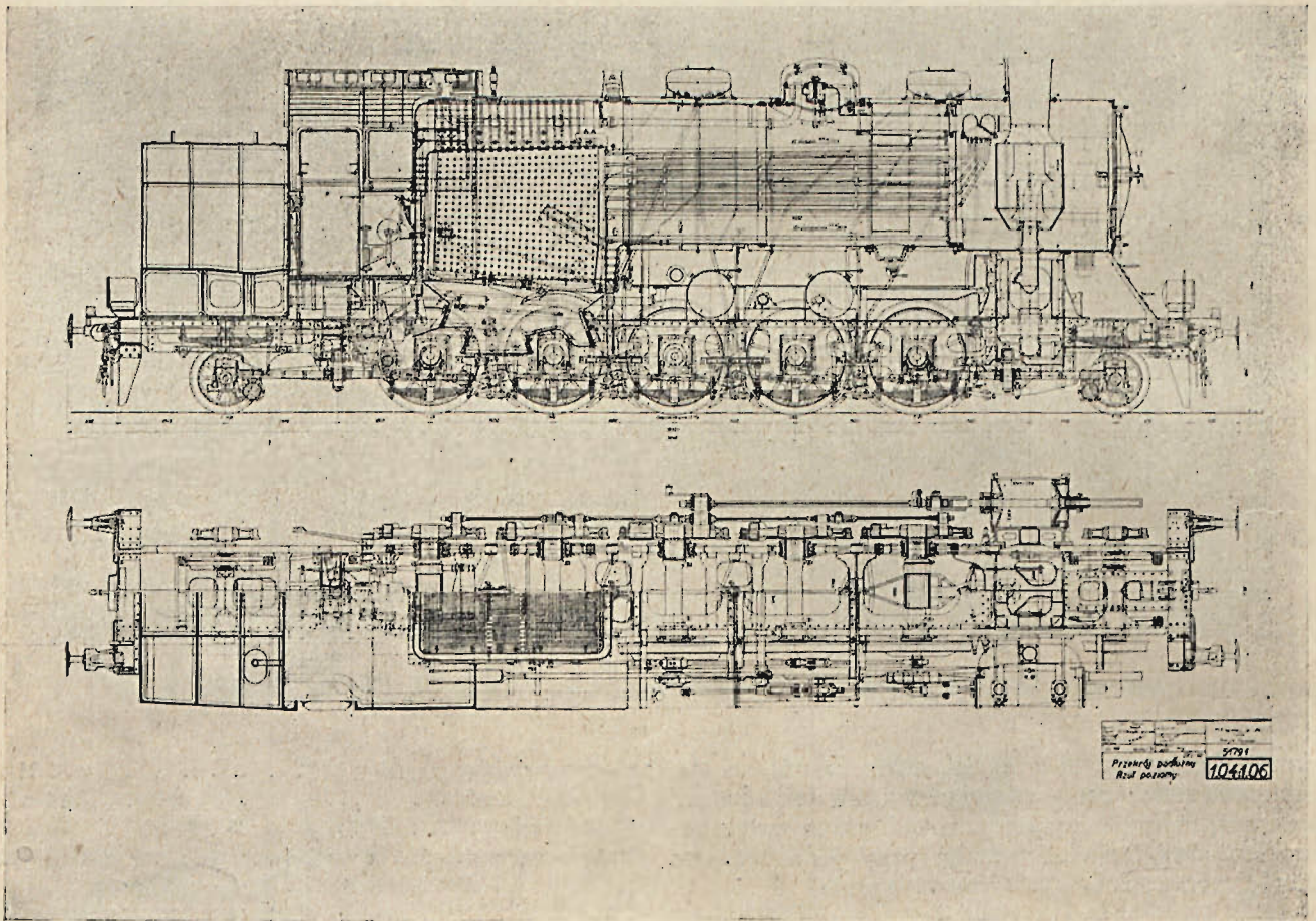
Rys. 2. Przekroje p0dłużne parowozu serii OKz32.
