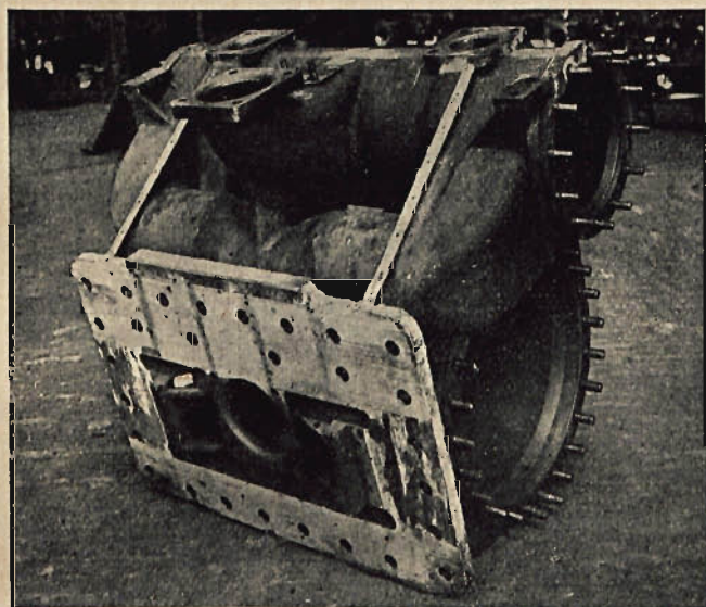
Rys. 6. Cylinder parowy parowozu serji OKz32
