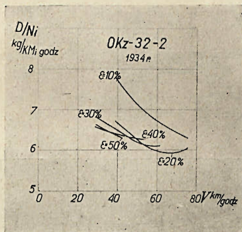
Rys. 8. Rozchód pary na 1 KM i godz. w zależności od zmiany napełnień cylindra i szybkości jazdy.
