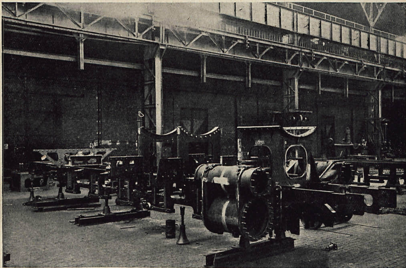
Rys. 3. Widok zmontowanego podwozia parowozu serii OKz32.
