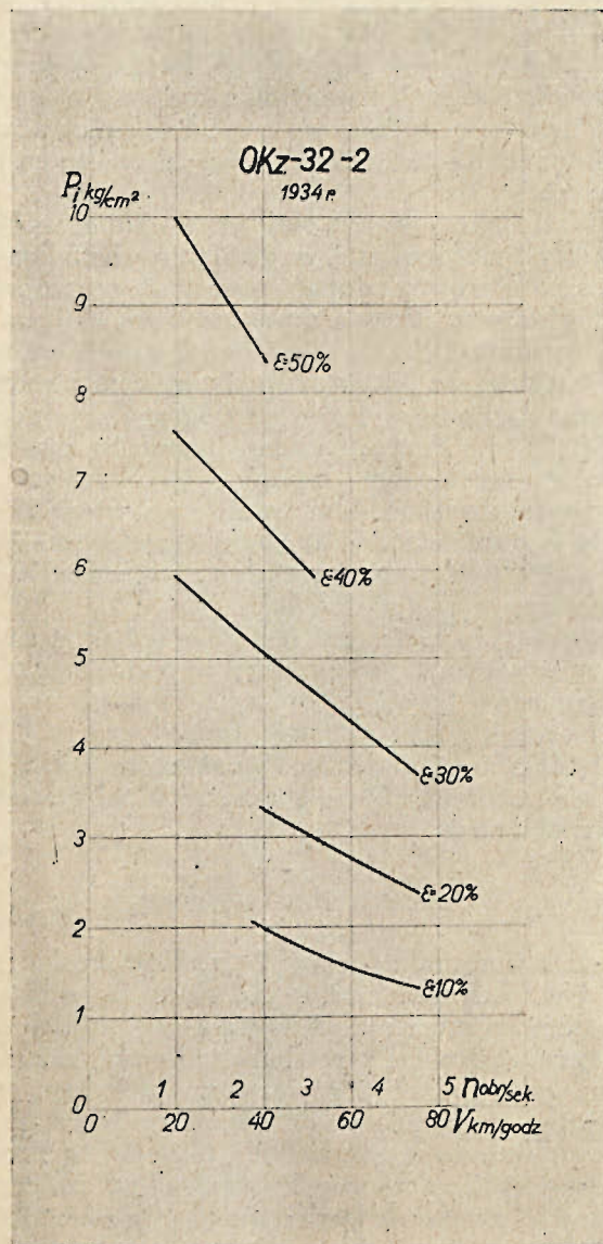
Rys 7. Ciśnienie indykowane w zależności od zmiany napełnień cylindra i szybkości jazdy.
