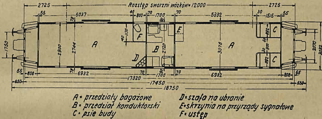
Rys. 1. Plan wagonu.
