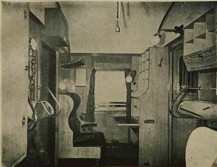
Rys. 4. Wnętrze przedziału konduktorskiego. Strona konduktora bagażowego.
