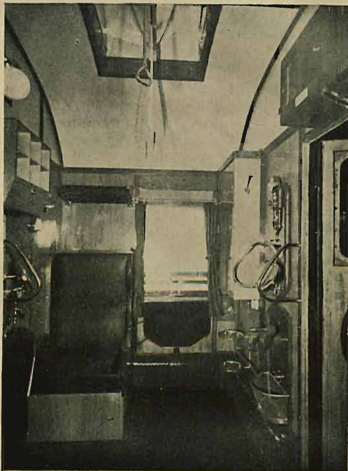
Rys. 3. Wnętrze przedziału konduktorskiego. Strona kierownika pociągu.
