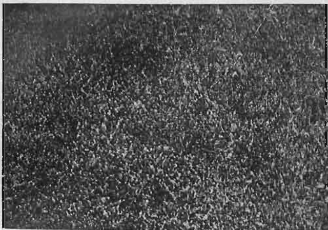
Rys. 7. Ulepszenie zastępcze doskonałe, struktura sorbityczna.
