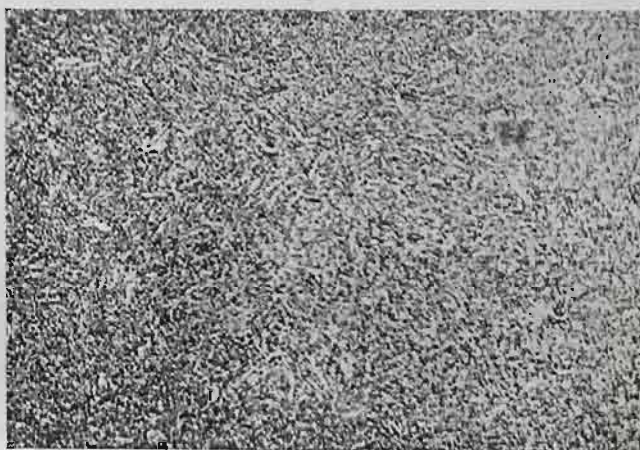
Rys. 5. Struktura sorbityczna, otrzymana przy termicznym ulepszeniu. (Szbk. hart. 50°/sek.)
