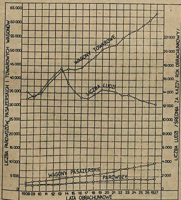
Fig. 4. Liczba jednostek taboru kolejowego i liczba ludzi w warsztatach.
