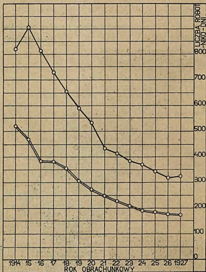
Fig. 3 a. Średnia liczba robotniko-dni potrzebnych dla naprawy jednego parowozu.
