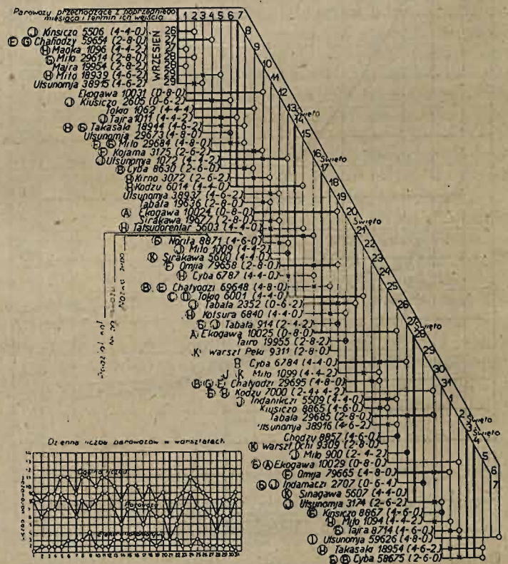
Tabl. III. Wykres wykonawczy wejścia i wyjścia parowozów. Październik 1928. Warsztaty Omija.
