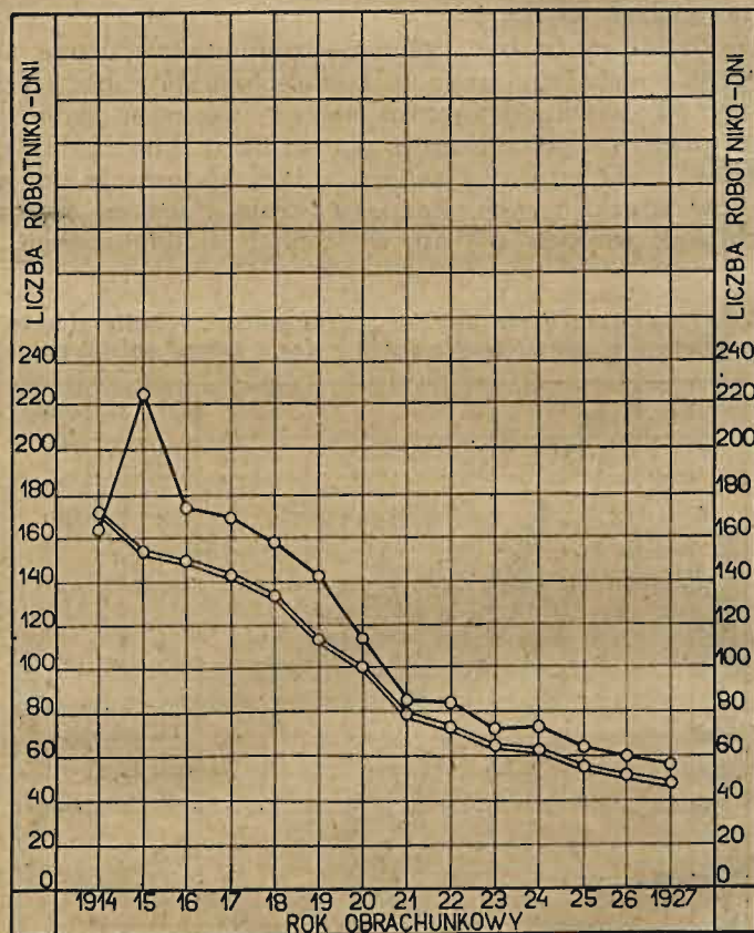
Fig. 3 b. Średnia liczba robotniko-dni potrzebnych dla naprawy jednego pasażerskiego wagonu.
