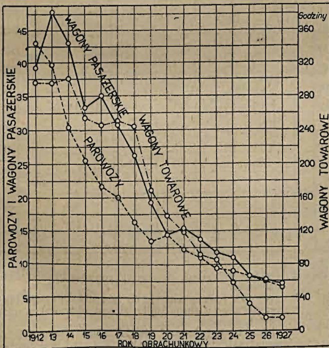
Fig. 1. Średnia liczba dni lub godzin potrzebnych dla głównej naprawy w warsztatach różnego rodzaju taboru kolejowego.
