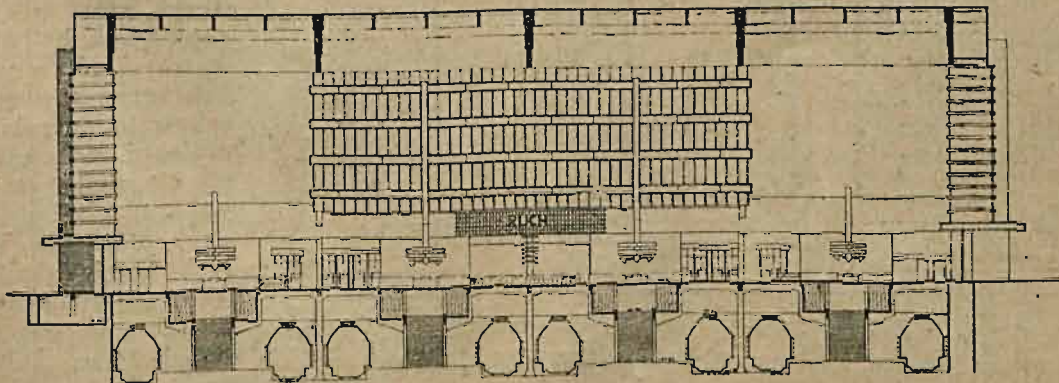
Przekrój poprzeczny 4-4 przez halę dla odjeżdżających.
