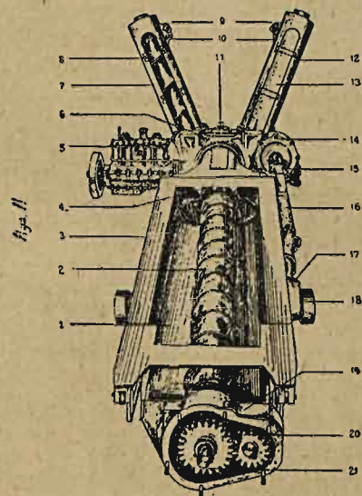
Części składowe mechanizmu podawacza węgla.
