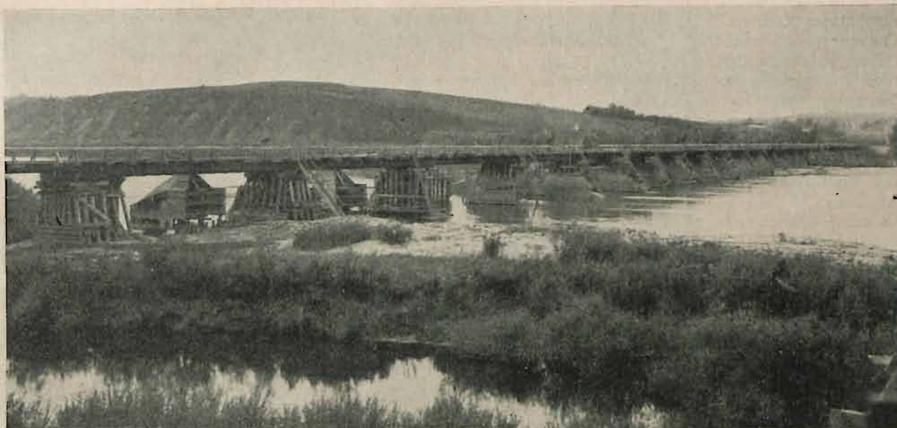
Budowa mostu kratowego żelaznego o śred. 75,00 m. X 6 na Wiśle pod Sandomierzem. Dawny most prowizoryczny.
