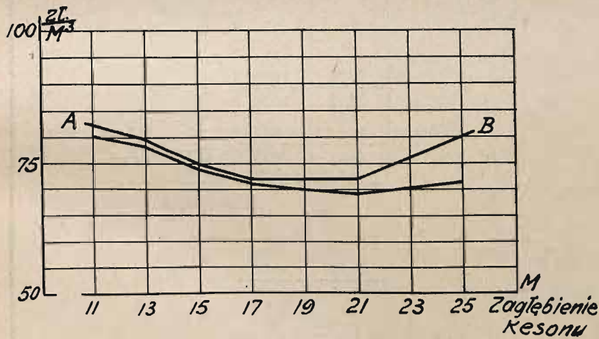
Koszt 1M 3 robót kesonowych
