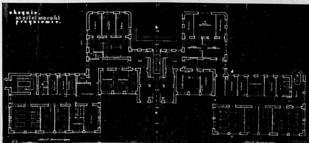
Rzut przyziemia 1:500.
