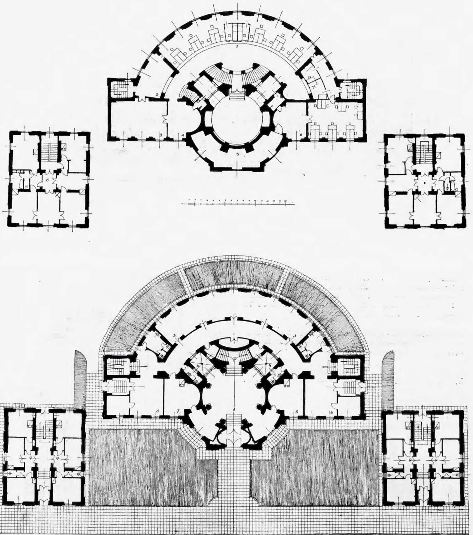
22 — 23. Arch. Marjan Lalewicz (Warszawa). Gmach Oddziału Banku Polskiego w Tomaszowie Mazowieckim. Rok 1924.
