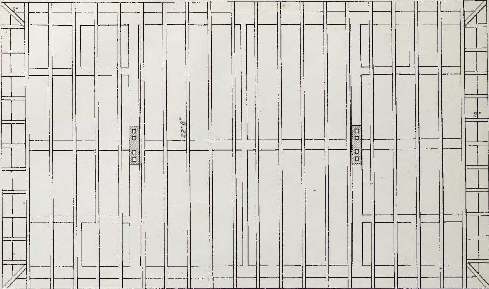
PLAN WIĄZANIA DACHOWEGO.
