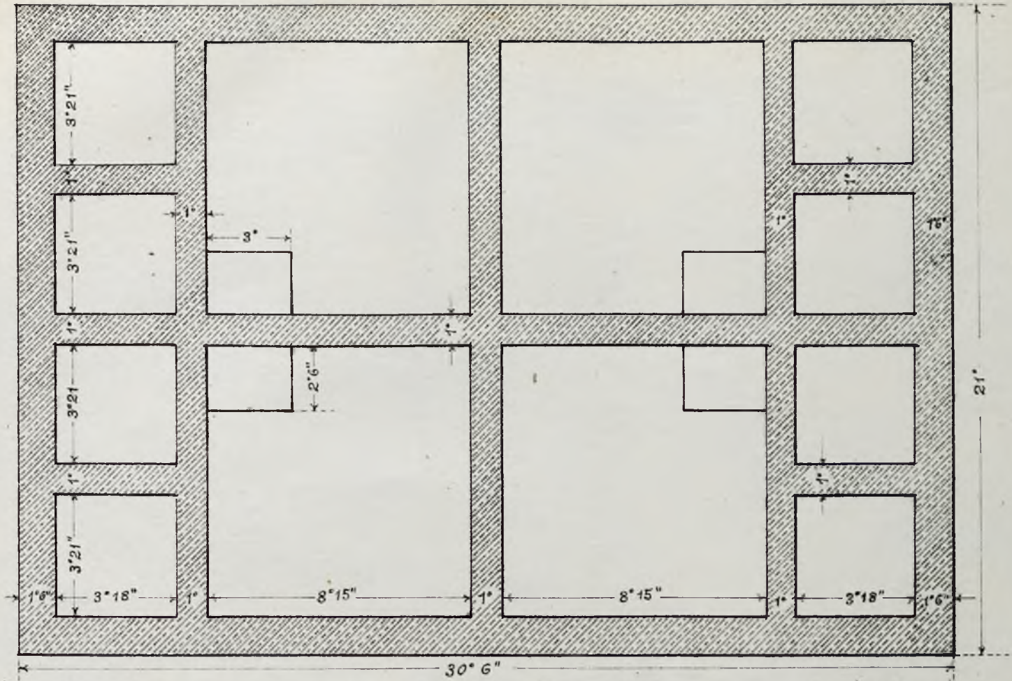
PLAN PARTERU.
