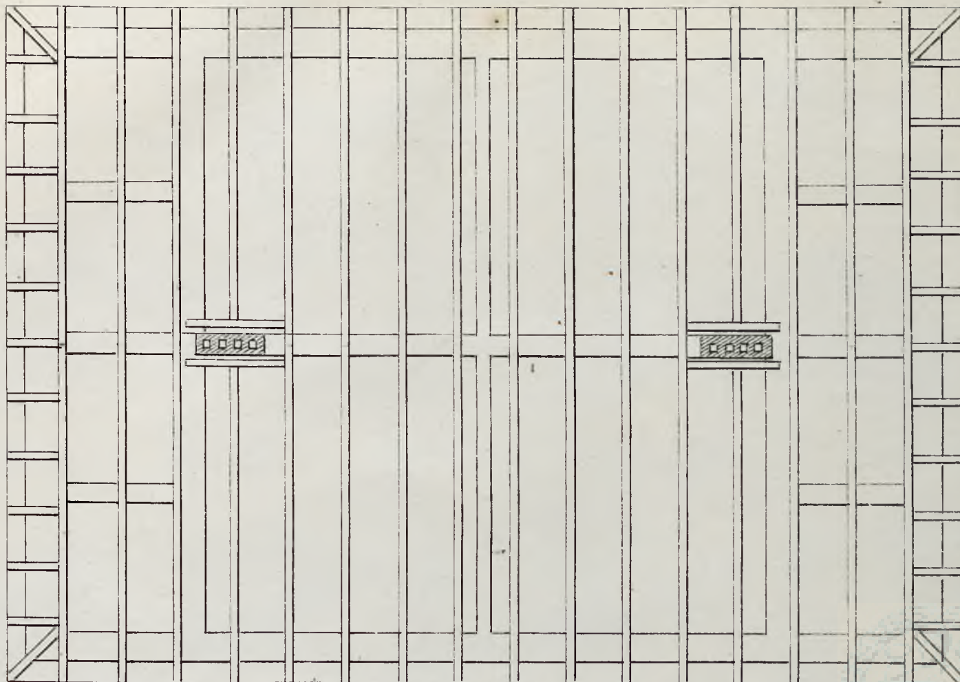
PLAN WIĄZANIA DACHOWEGO.
