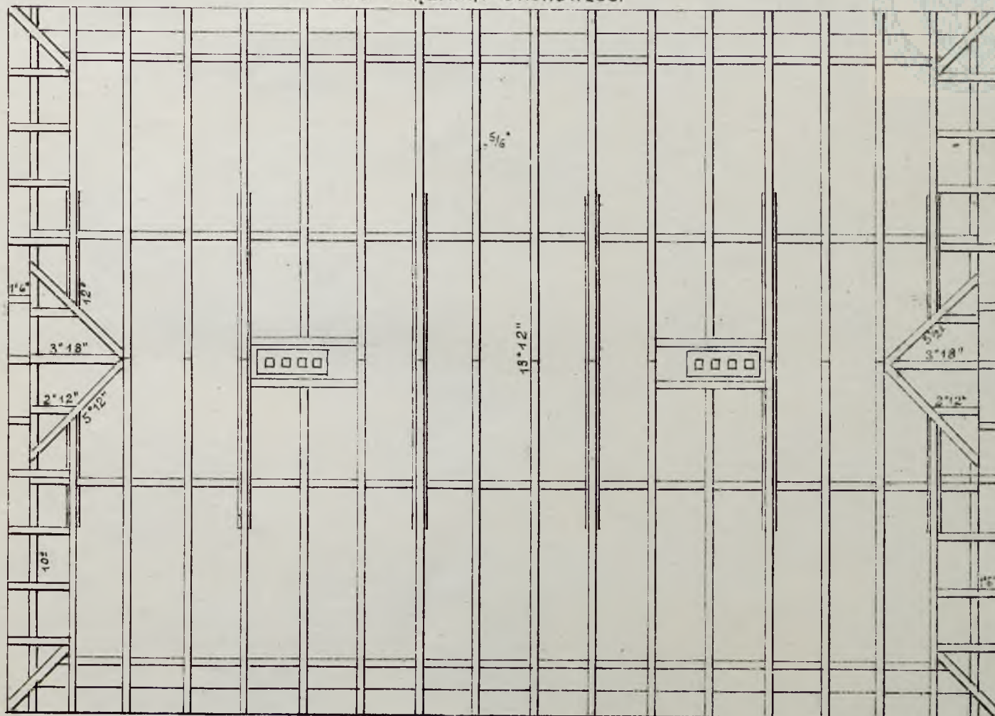
PLAN WIĄZANIA DACHOWEGO.
