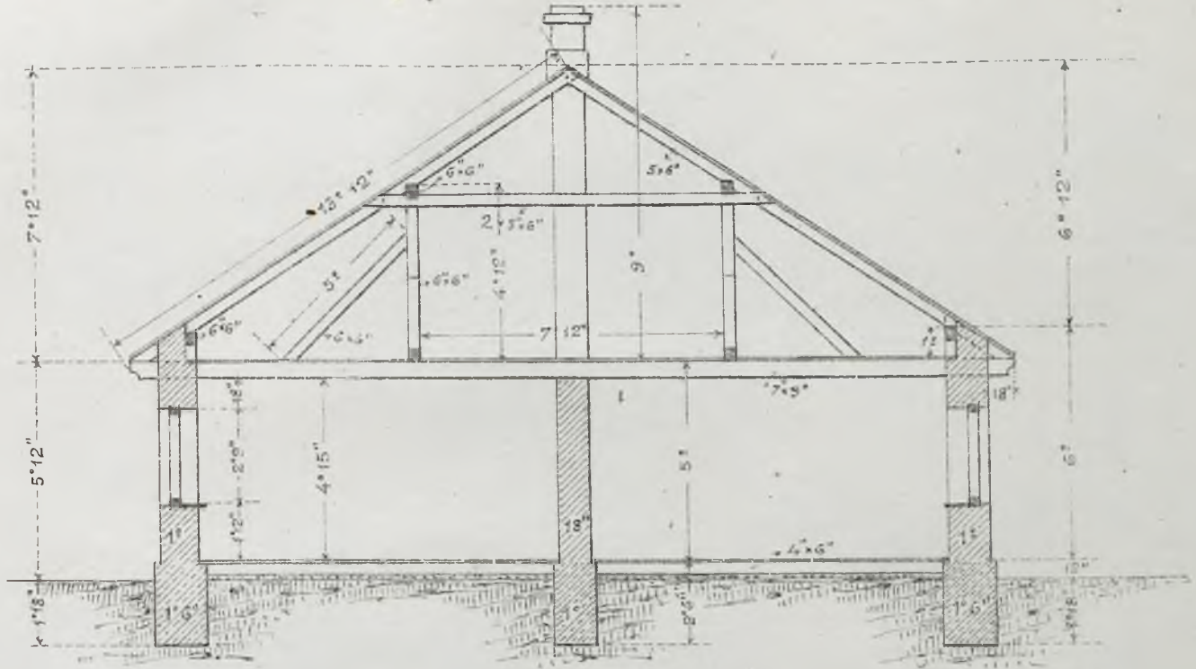
PRZEKRÓJ POPRZECZNY.
