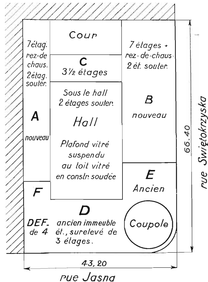
Fig. 2 — Plan de l'ensemble. Plan gmachu.
