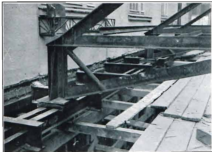
Fig. 104 Fig. 104. — Pied d'une ferme. Stoпа więzara.
