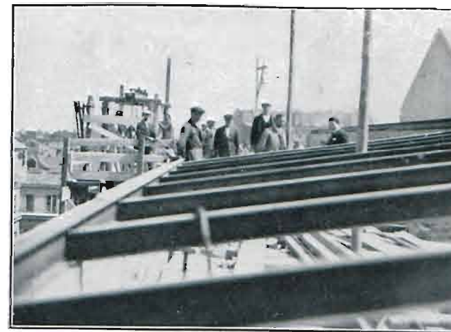
Fig. 32 Construction du toit de la partie A. Dach spawany oficyny A., wykonany z dwuteowników.
