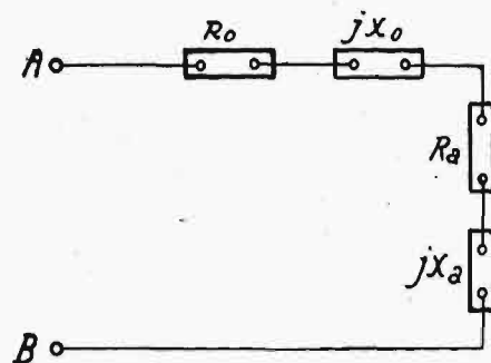
Rys. 4. Schemat zastępczy głośnika.
