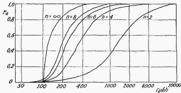
Rys. 14. Opór promieniowania dla tub o różnej krzywiźnie.
