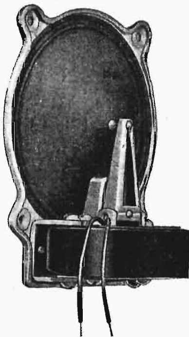
Rys. 9. Głośnik z przekładnią mechaniczną i-my „The Best Manufacturing Company”.
