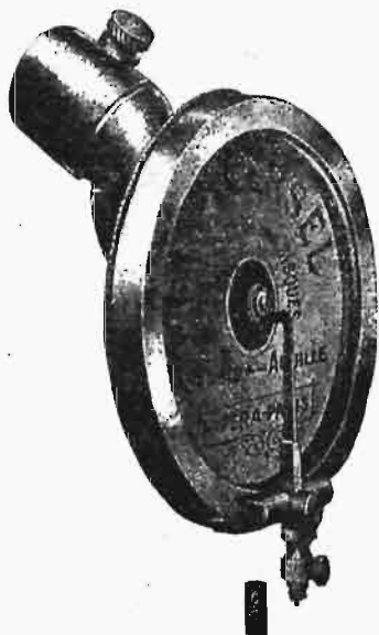
Rys. 8. Membrana gramofonowa z przekładnią mechaniczną.
