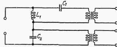
Rys. 19. Schemat filtru do zespołu dwugłośnikowego.
