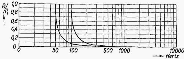
Rys. 16. Odbicie energii przy wylocie tuby wykładniczej.
