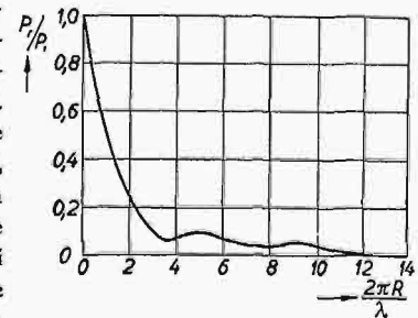
Rys. 15. Odbicie energii przy wylocie rury cylindrycznej.
