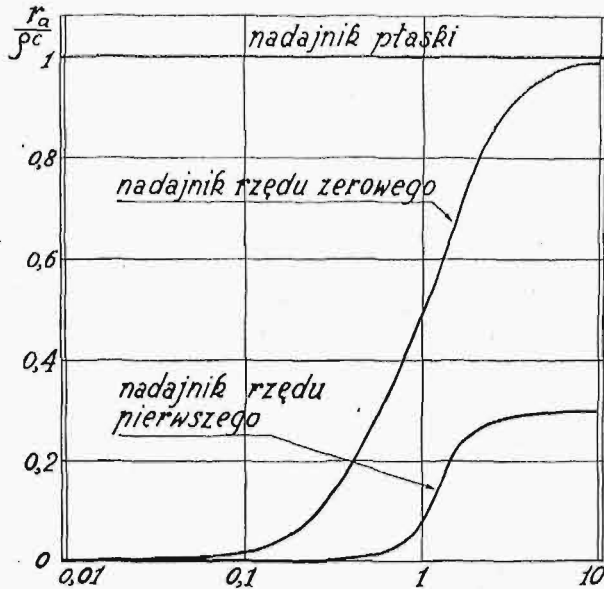
Rys. 5. r_a = f(\xi) dla różnych nadajników teoretycznych.
