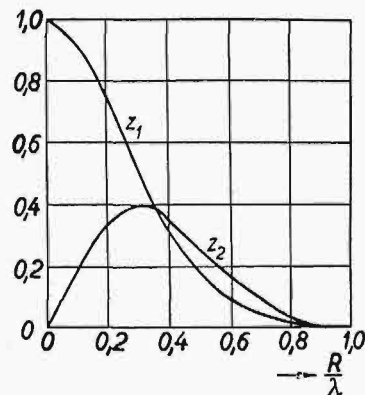
Rys. 11. Zniekształcenia linijowe w przekładni akustycznej.
