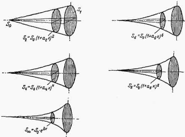
Rys. 13. Tuby o różnej krzywiźnie.
