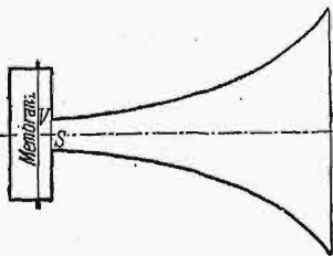
Rys. 17. Schemat pierwotnego głośnika tubowego.
