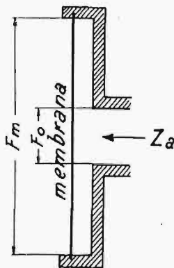
Rys. 10. Schemat prymitywnej przekładni akustycznej.
