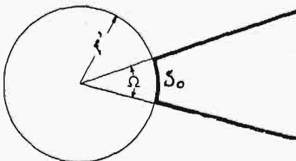
Rys. 12 Zasada działania tuby stożkowej.
