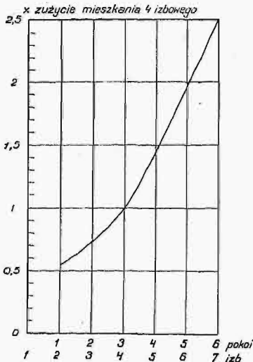
Rys. 2. Zużycie energii el. mieszkania różnej wielkości przy założeniu, że zużycie mieszkania 4-izbowego = 1 (Rohrbeck).
