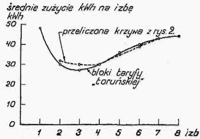
Rys. 3. Średnie zużycie, przyjęte za podstawę wysokości I bloku taryfy „toruńskiej” w porównaniu z przebiegiem średniego zużycia, stwierdzonego dla 14 elektrowni niemieckich.
