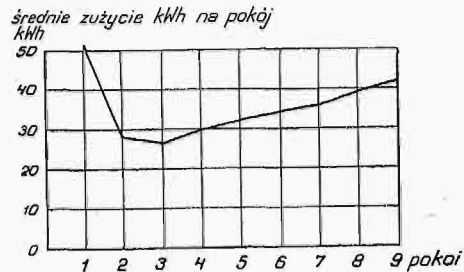
Rys. 4. Średnie zużycie energii el. na pokój według przeciętnej 36 taryf niemieckich (Vogl).
