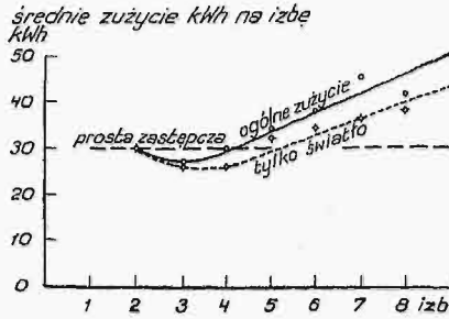
Rys. 1. Średnie zużycie energii el. na izbę dla mieszkań w Toruniu (P. E. 1932, str. 654).
