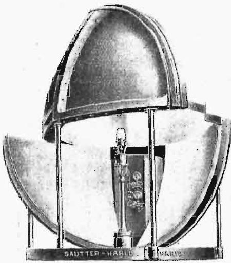
Rys. 5. Latarnia lustrzana czterosegmentowa o lustrze metalowym w Galiton (Tunis).
