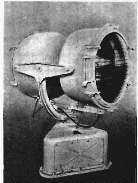
Rys. 4. Lustrzana latarnia lotnicza firmy amerykańskiej „Aga” o podwójnym systemie optycznym.
