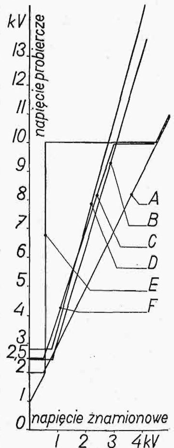
A—CEI 2U+1000, B—Niemcy, olej, suche na gorąco, C—Polska propozycja, D—Niemcy, suche — na zimno, E—CEI Transf. publiczne, F—3,25 U.
