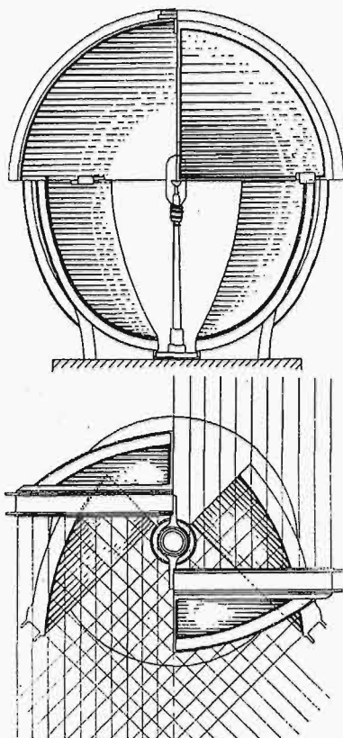
Rys. 8. Układ wiązek świetlnych latarni segmentowej, dającej dwie grupy, złożone z 1-go i 3-ich błysków.
