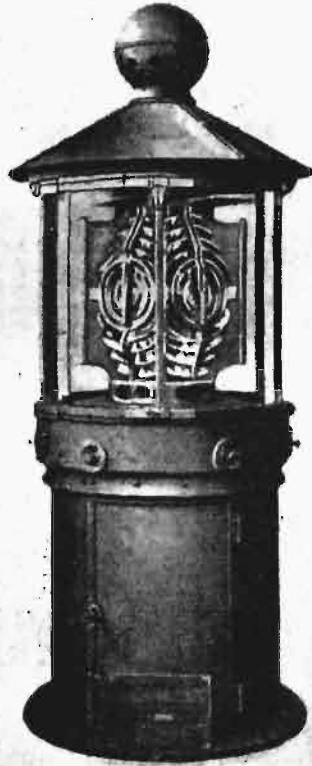
Rys. 3. Latarnia lotnicza dioptryczno-katadioptryczna, zastosowana na lotniskach we Lwowie, Katowicach i Poznaniu.
