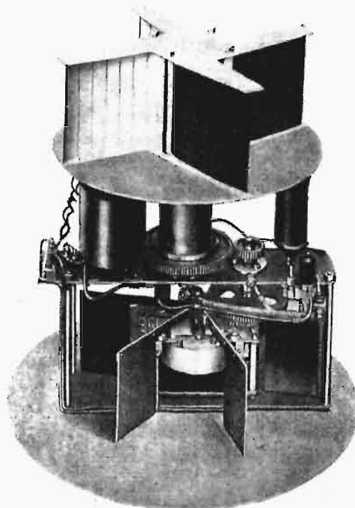
Rys. 10. Latarnia lotnicza lustrzana 4-błyskowa, wyyskująca prawie w całości źródło światła.
