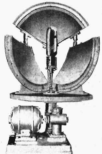
Rys. 7. Latarnia trójbłyskowa o lustrach szklanych.
