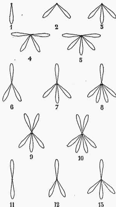
Rys. 9. Zestawienie układów błysków, stosowanych w nowoczesnych latarniach lustrzanych (pojedyncze grupy błysków od 1 do 5; od 6 do 13 podwójne grupy błysków, złożone z jednego lub dwu błysków oraz z jednego, dwu, trzech i czterech błysków).
