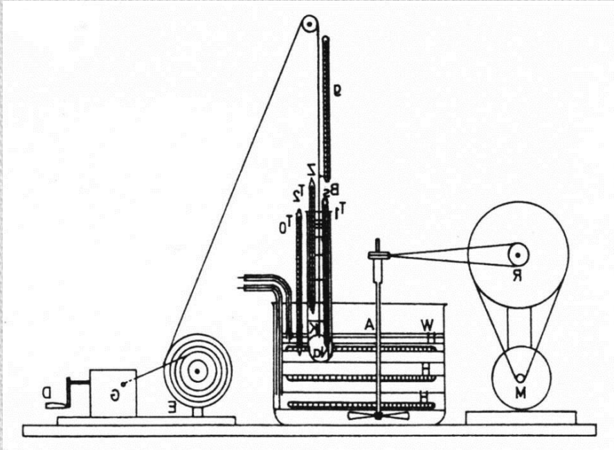
Rysunek z pracy J. Czochralskiego pomiar szybkości krystalizacji sodu.
