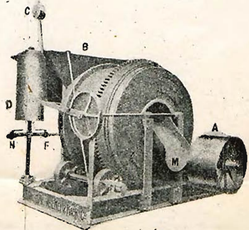
Rys. 112. Betonierka Ransoma.
