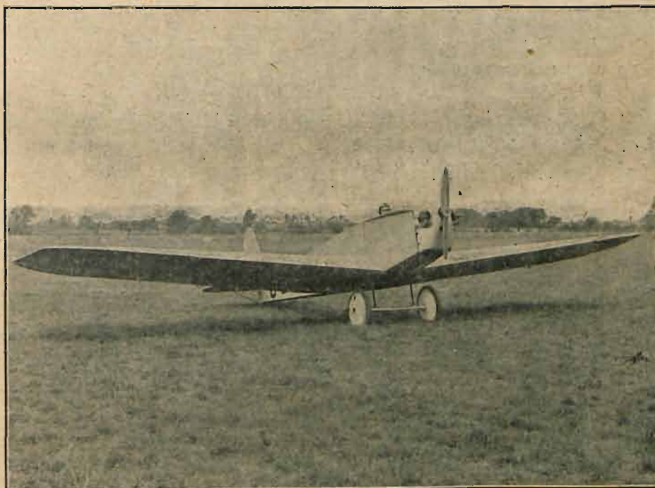
Płatowiec sportowy „BRISTOL“ jeden z zwycięzców konkursu w Lympe w Anglii. Silnik 14. KM. Płatowiec ten osiąga wysokość 1500 mtr. w 14 minutach i posiada szybkość 135 km na godzinę. Jak to widać z fotografii posiada zwyczajny silnik motocyklowy.
