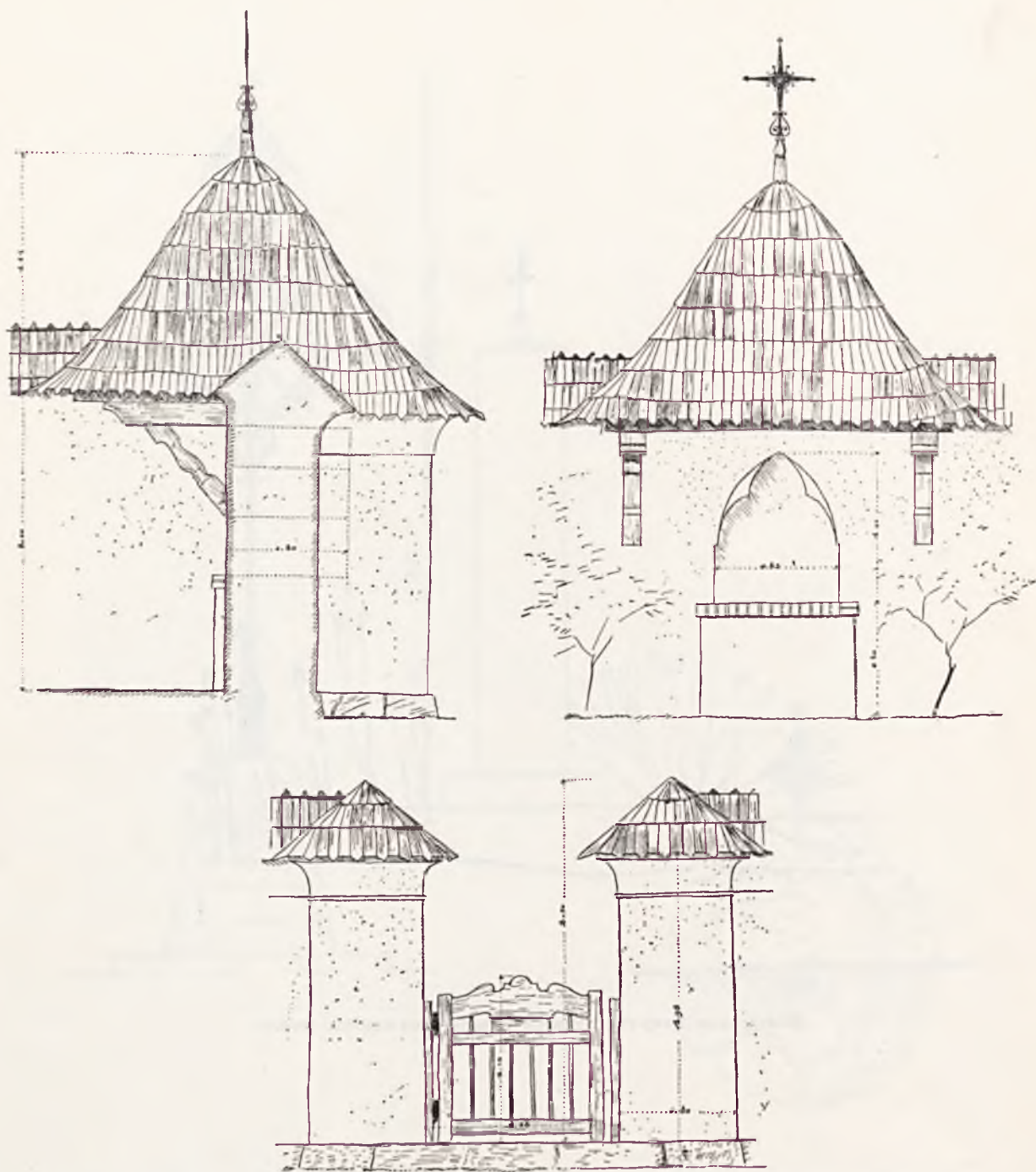
Romuald Gutt: Szczegóły ogrodzenia cmentarzyka wojennego. Nagroda I.
