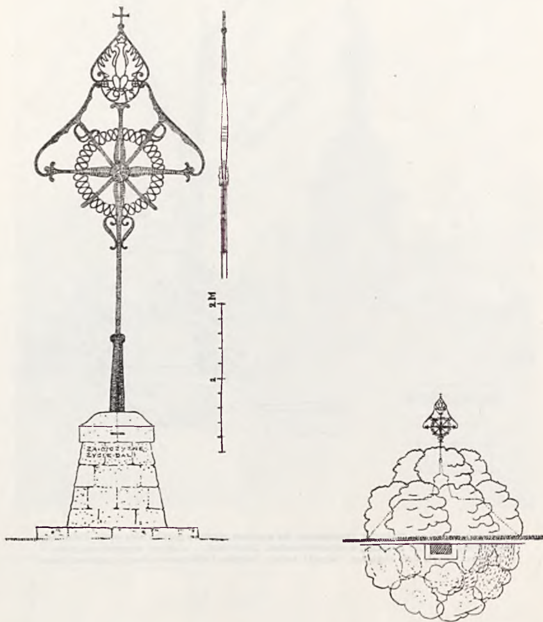
Zygmunt Harland: Krzyż żelazny kuty — na podstawie kamiennej, ustawiony na kurhanie mogilnym 2.50—3.00 m. wysokości. Krzyż projektowany jako pamiątka walk Legionów. Kurhan zasadzony krzewami typowymi dla danej okolicy. Krzyż winien być ustawiony na wysokim miejscu — by nie mleć tła za sobą. Projekt wyróżniony.
