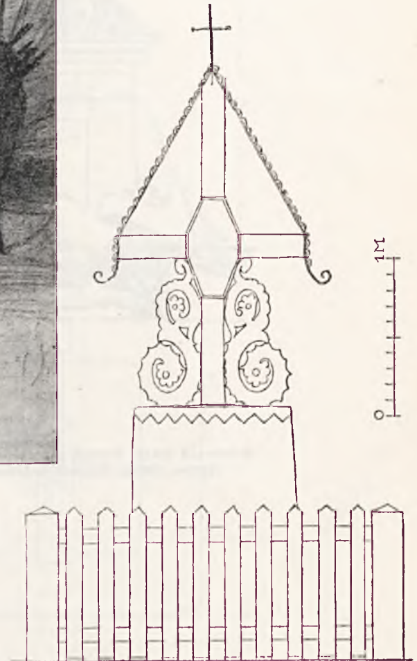
Józef Seredyński: Na cokole murowanym z cegły lub kamienia polnego osadzony krzyż drewniany z drewnianą wycinanką z szerokiej deski twardego drzewa. Na skrzyżowaniu ramion krzyża tablica drewniana, na której ma być umieszczony napis cięty lub też nabita tabliczka z nazwiskiem i datą. Nad ramionami krzyża rodzaj dachu z blachy, na cokole okrycie blachą chroniące od zaciekania. Ogrodzenie drewniane. Projekt zakupiony przez Muzeum Techniczno-przemysłowe w Krakowie.
