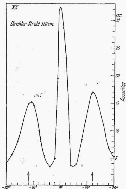
Rys. 2. „Direkter Strahl” oznacza natężenie wiązki pierwotnej. Wiązce odbitej odpowiada tylko ok. 32 cm., t. j. wiązka ta zawiera ok. 0,1 całkowitej liczby cząsteczek. Każdej z dwóch wiązek ugiętych odpowiada ok. 17 cm.
