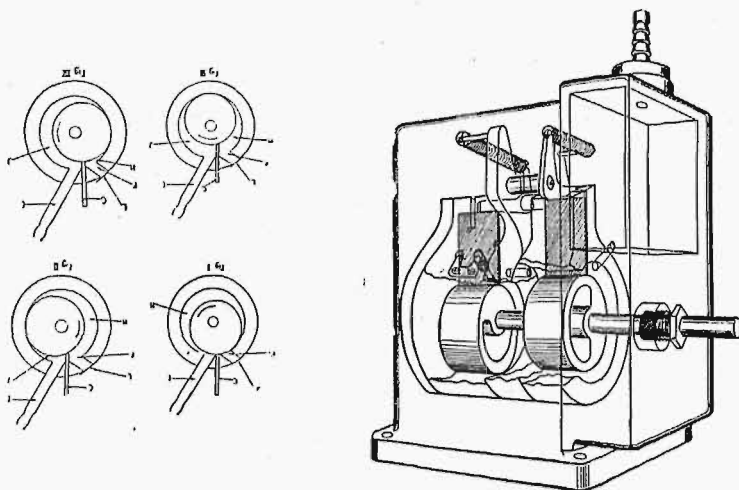
Rys. 2. Z lewej strony — 4 fazy całkowitego obro'u rotora. Z prawej strony — przekrój perspektywiczny pompy.
