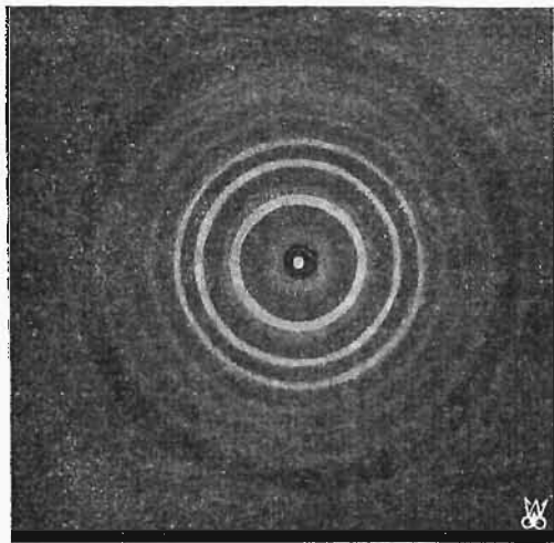
Rys. 5. Röntgenogram cystyny, substancji złożonej z nieuporządkowanych krystalitów.
