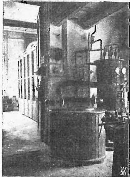
Rys. 5. Maszyna chłodnicza, „Tiefkühler“ i komory termiczne.
