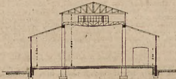
Przekrój poprzeczny.
