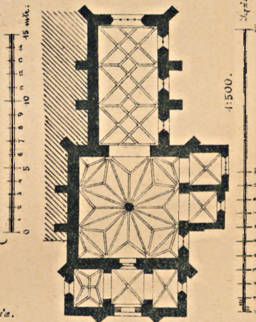
Rys. 2. Kościół Sgo Kiriak w Strakonice. (W dzisiejszym stanie)
