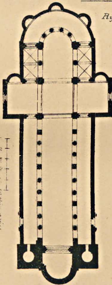
Rys. 5. Rzut poziomy kościoła S. Gotthardt w Hildesheim.
