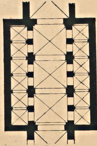
Rys. 2. Pierwotny, domniemywany system sklepienny kościół w Mogilnie. (Podług W. Luszczykiewicza - Sprawozdania kom. do badania hist. sztuki w Polsce.)
