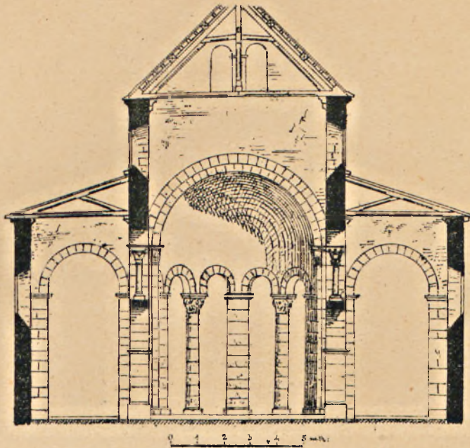
Rys. 1. Przekrój kościoła w Vignory. (Viollet-le-Duc.)
