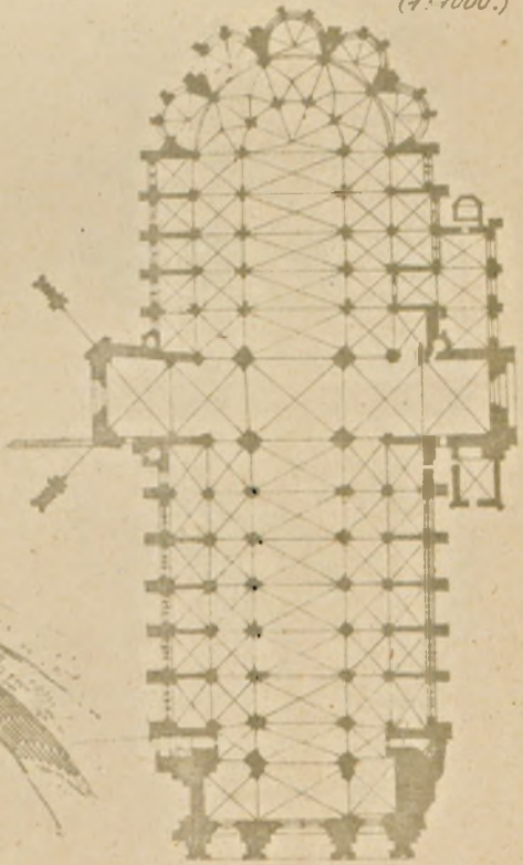
Rys. 3. Katedra w Tours. 1:1000.
