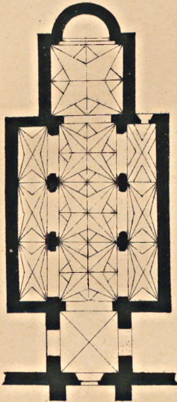
Rys. 1. Rzut poziomy kościoła klasztornego (Benedyktynskiego) w Mogilnie. (Wiek XII.)
