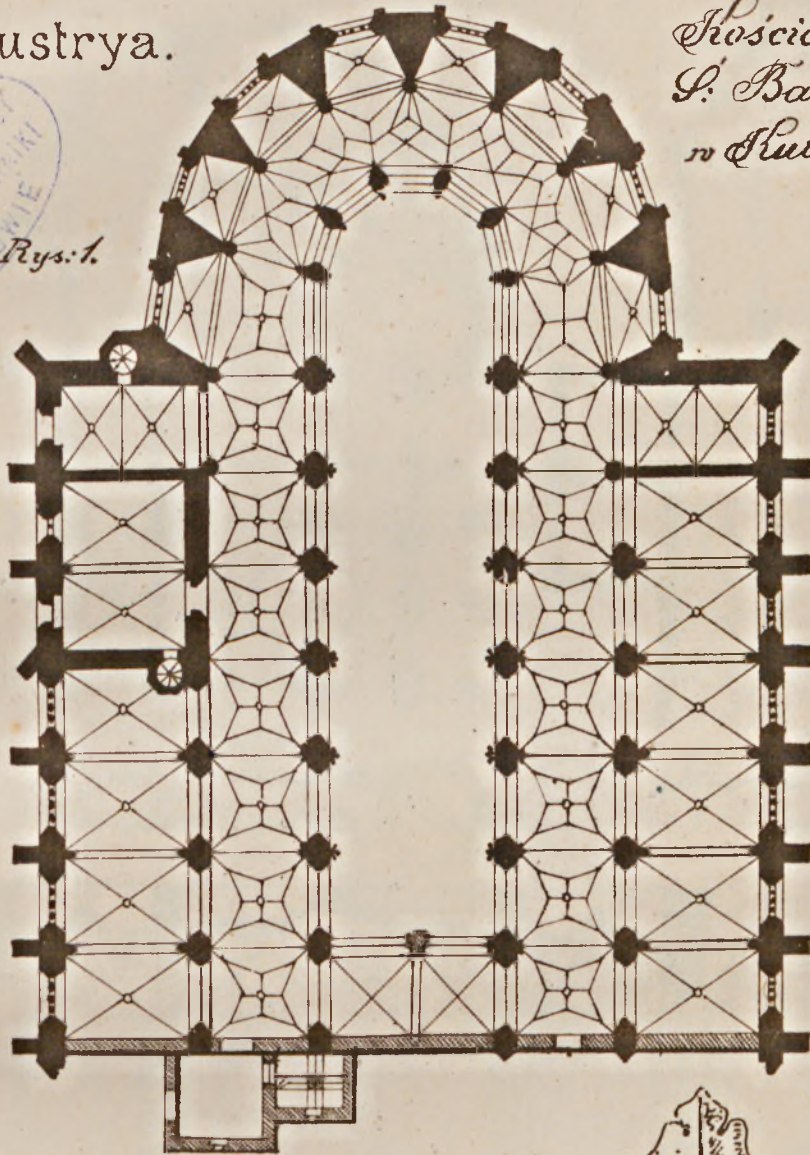
Ornament z tuku odpornego kości. Ś. Barbary w Sluttenberg.
