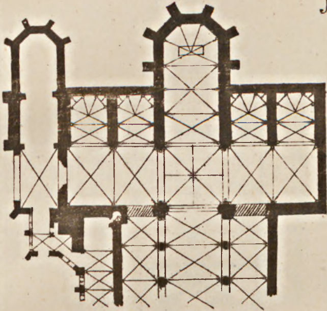
Rys. 1. Chór kościoła klasztornego „Las Huelgas” koło Burgos.
