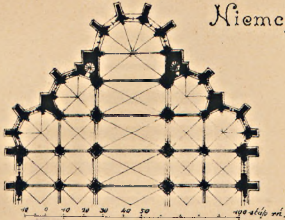
Rys. 1. Świątynia w Xanten.
