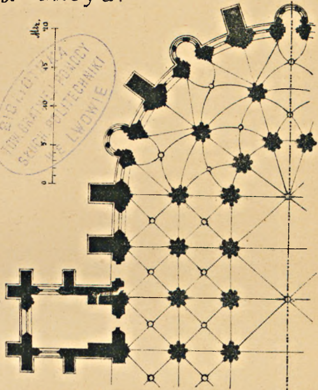
Rys. 2. Chór katedry w Bourges. (1230)
