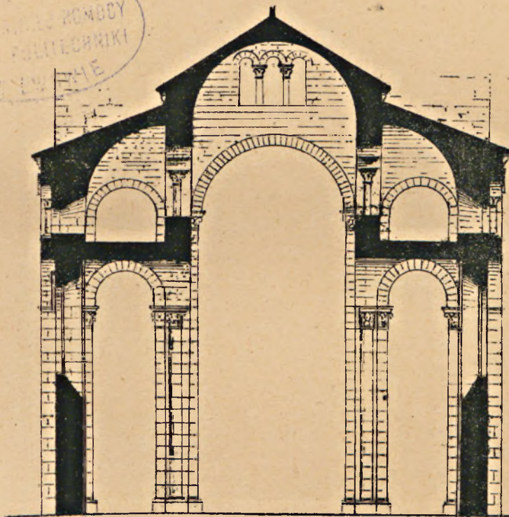
Rys. 3. Przekrój poprz: kościoła „Notre Dame du Fort” w Clermont. (Viollet-le-Duc.)
