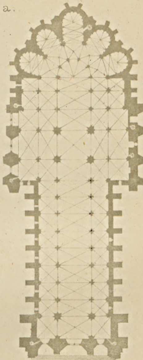
Rys. 2. Katedra w Reims. (0,001 m - 1mtr.)
