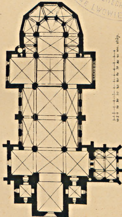
Rys. 6. Rzut poziomy kościoła katedralnego w Münster.
