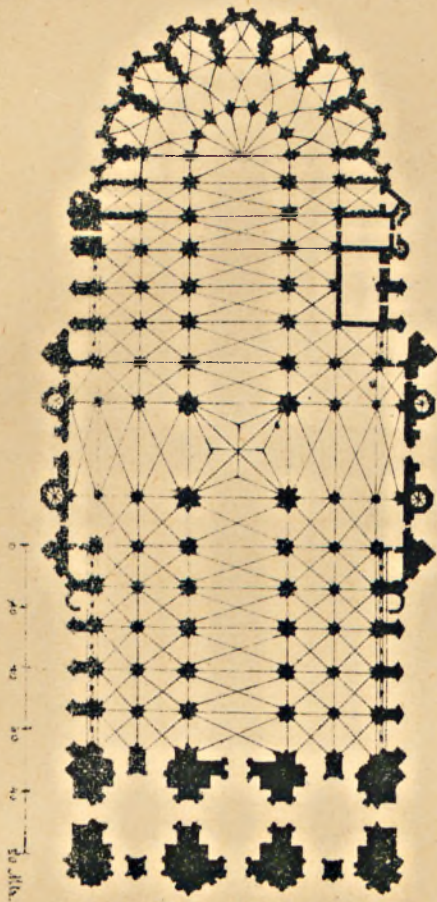
Rys. 1. Katedra w Orleanie.
