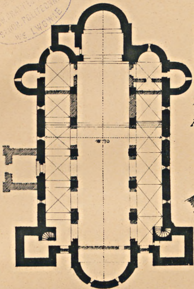
Rys. 1. Plan poziomy kościoła w Łęczycy, dziś we wsi Turmie. (M. w.)
