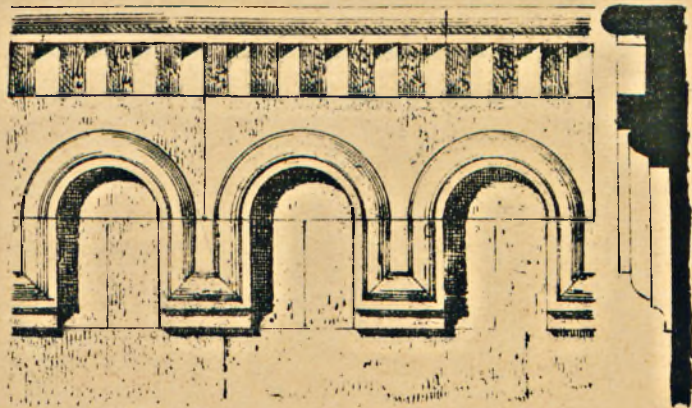
Rys. 4. I kościoła w Sönggrabern. (Austryca) (do Tabl. XXVII.)
