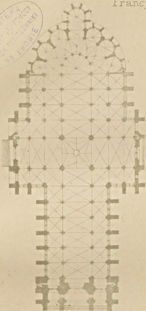
Rys. 1. Katedra w Amiens. (1:1000.)
