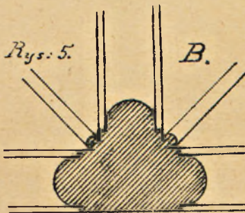
Rys 3. Część przekroju podłużnego kościoła „St. Maria del Carmine. (Włochy) Rys 4. 5. i 6. szczegóły do rys 3go. (Do Tabl. XXXI)
