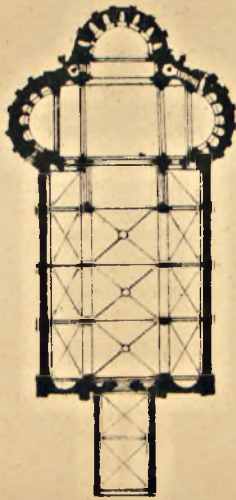
Rys. 1. Kościół podwójny w Schwarz-Rheindorf.
