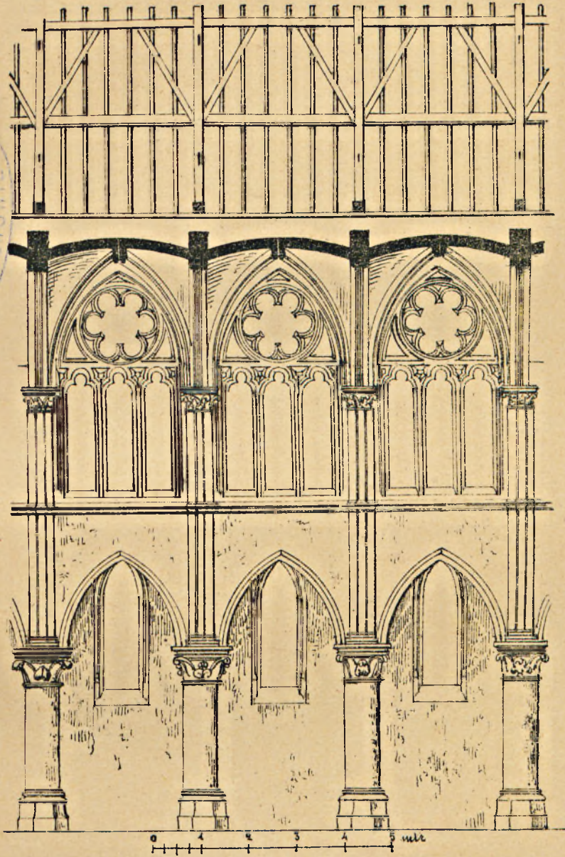
Przekrój podłużny kościoła w Champagne.
