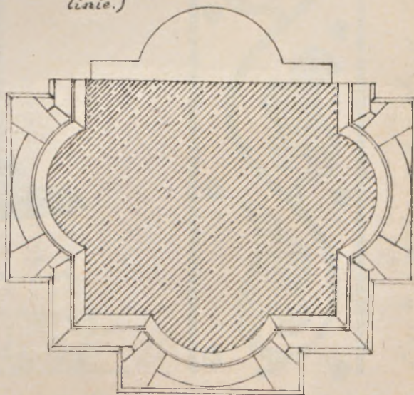
Rys. 5. Krut poziomy filaru międzynawowego w kościele w Sulejowie.
