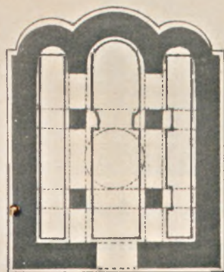
Rys. 2. Cerkiew Sgo Spasa w Łańcutu, pod Haliczem. (Fundamenta oznaczają grubsze linie.)
