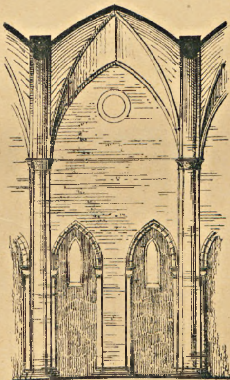
Rys 3. Część przekroju podłużnego kościoła „St. Maria del Carmine. (Włochy) Rys 4. 5. i 6. szczegóły do rys 3go. (Do Tabl. XXXI)
