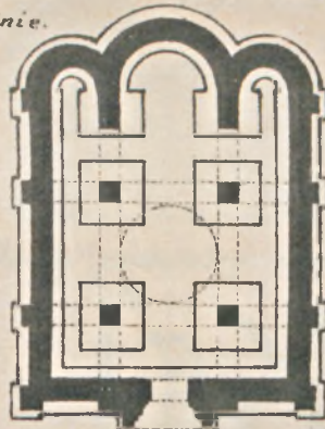
Rys. 3. Cerkiew Soga Rodzicy w Ła, Łańcut. (Fundament oznaczają grubsze linie.)
