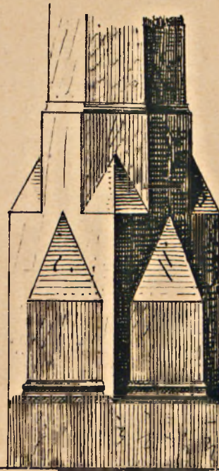
Podstawa słupa z drewna dębowego w Monachium.
