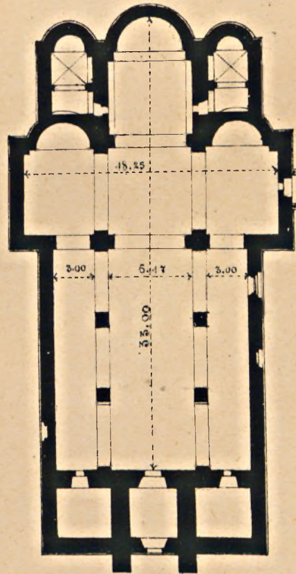
Rys. 4. Rzut poziomy kościół Ś. Józefa i Pawła w Huszowie.
