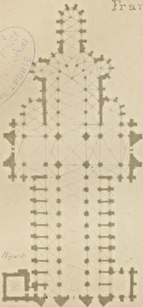
Katedra w Rouen. (1:1000)
