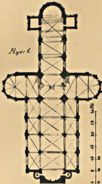
Plan tumanu w Bonn.
