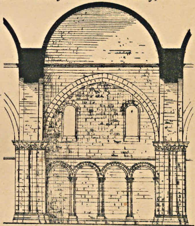
Rys. Słocień „St. Front” w Périgueux. (Przekrój). ~
