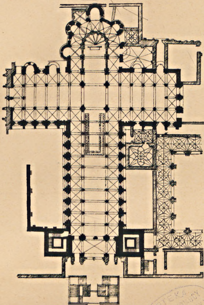
Rys. 1. Rzut poziomy katedry w Santiago de Compostella. (Hiszpania.)
