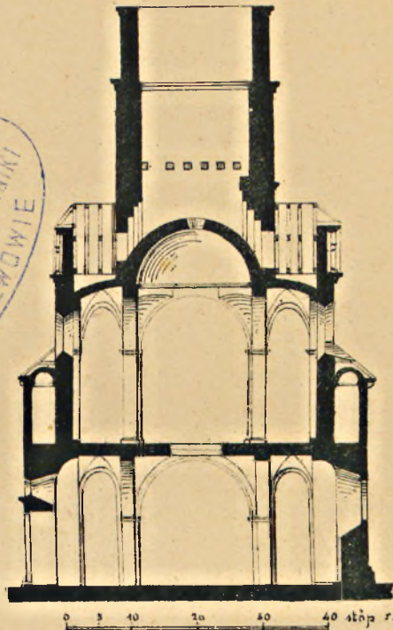
Rys. 2. dorys. Przekrój poprzeczny. ~
