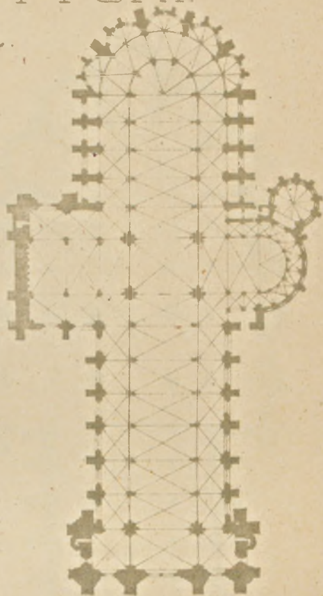
Rys. 2. Katedra w Poissons. (1:1000.)
