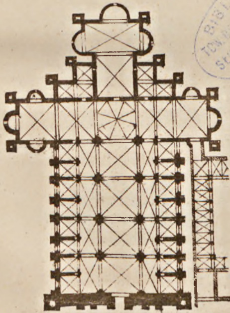
Rys. 3. Certosa w Pawi.
