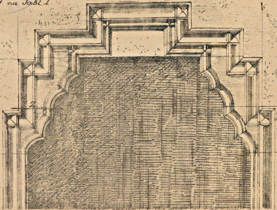
Rys. 2. Drzwi wchodowe z klasztoru S. Katarzyny w Strakowie. Okrój Z. przedstawia rys. 7 na Tabl. I.
