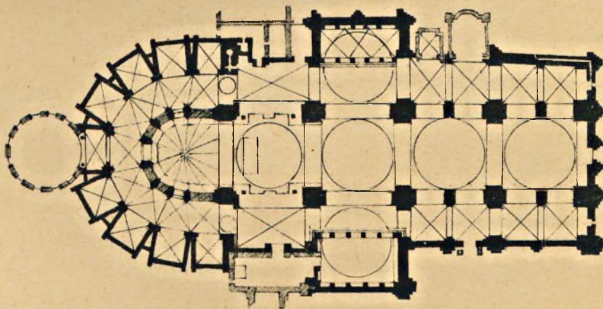
Rys. 3. Rzut poziomy kościoła Świętego Antoniego w Padwie.
