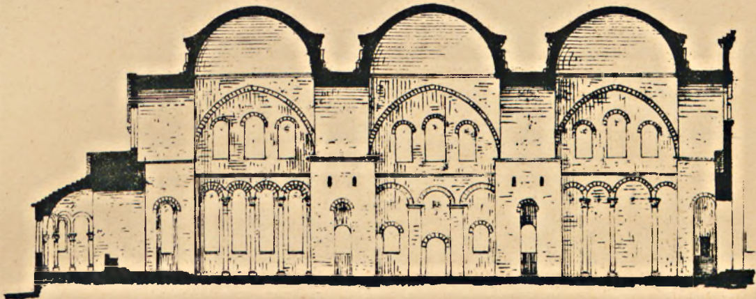
Rys. Słocień „St. Front” w Périgueux. (Przekrój). ~
