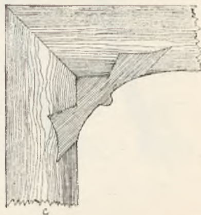
Ryc. 100 a-c. Więzby różne.
