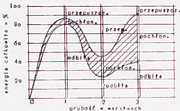
Rys. 9. Przechodzenie głosu przez 3 warstwy fileu grubości ca 6,5 mm.
