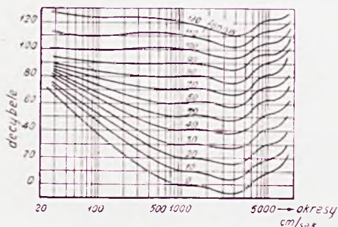
Rys. 7. Zależność między głośnością i natężeniem dźwięku.
