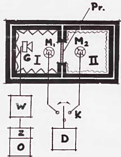
Rys. 11. Aparatura do mierzenia izolacji akustycznej.
