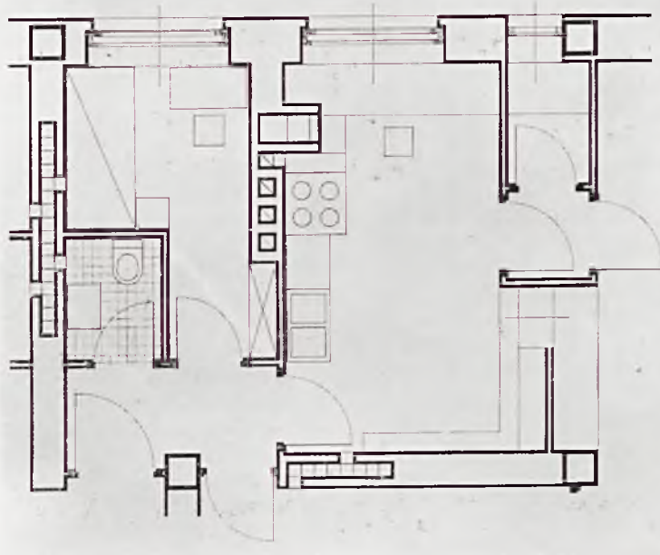
Plan części gospodarczej \frac{1}{20} powierzchnia 30 m 2
