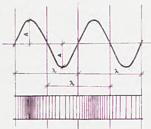
Rys. 1. Fale zgęszczenia i rozszerzenia i ich okres.
