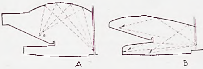
Rys. 3. Przekroje sali.
