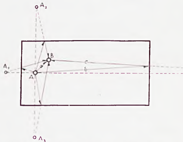
Rys. 2. Studium geometryczne odbicia głosu w sali najprościej.
