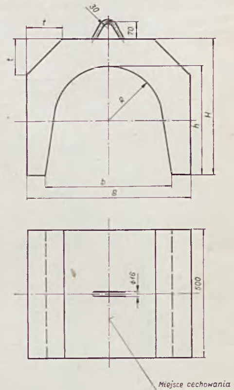
Rys. 1. Obciążnik siodłowy
