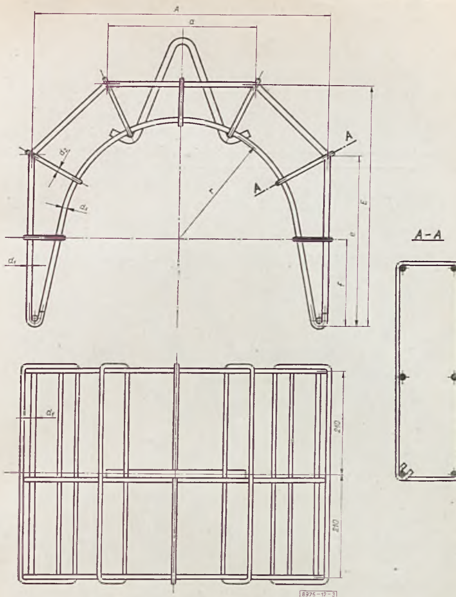
Rys. 3. Zbrojenie obciążników S-250 ÷ S-400
