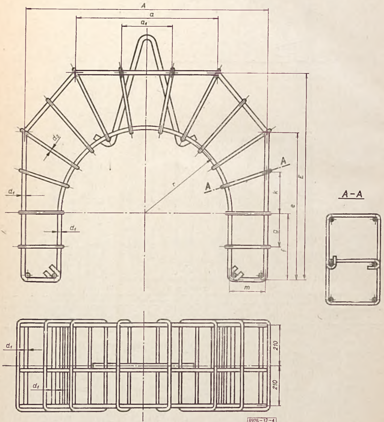
Rys. 4. Zbrojenie obciążników S-500 ÷ S-900
