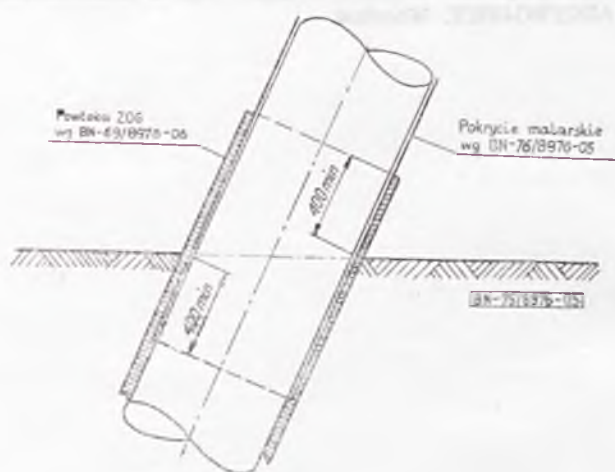
Łączenie pokryć malarskich z powłokami asfaltowymi
