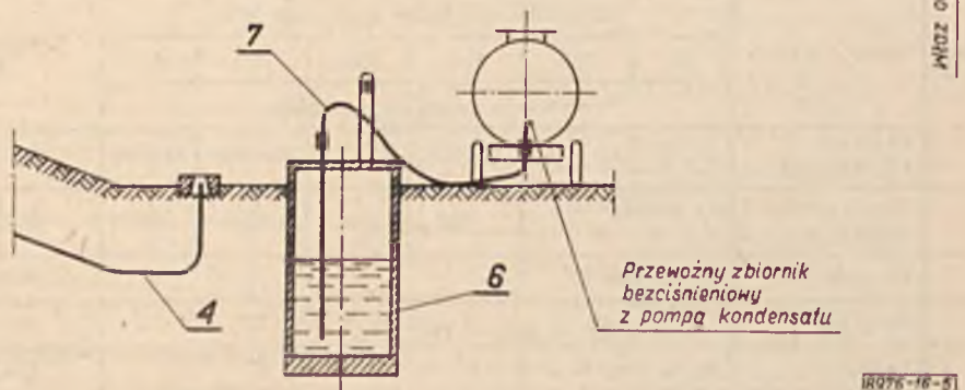
Rys. 5. Instalacja dwururowa z rurociągiem i zbiornikiem kondensatu
