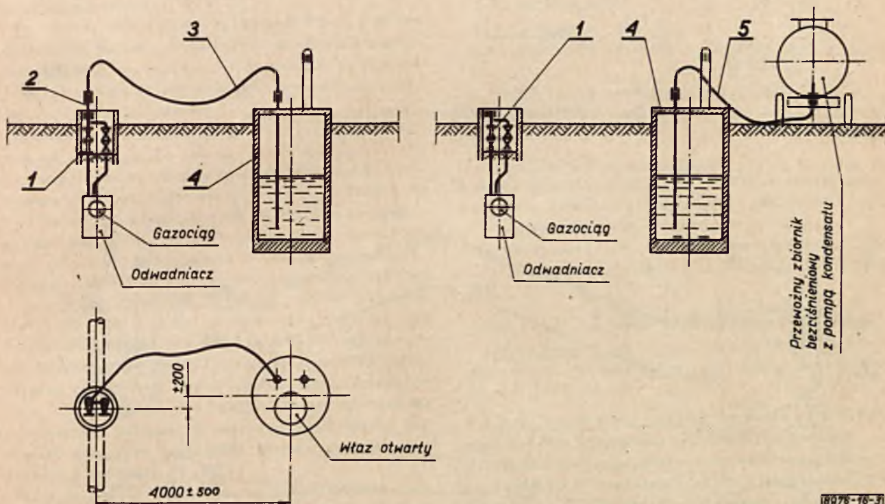
Rys. 3. Instalacja dwururowa ze zbiornikiem kondensatu
