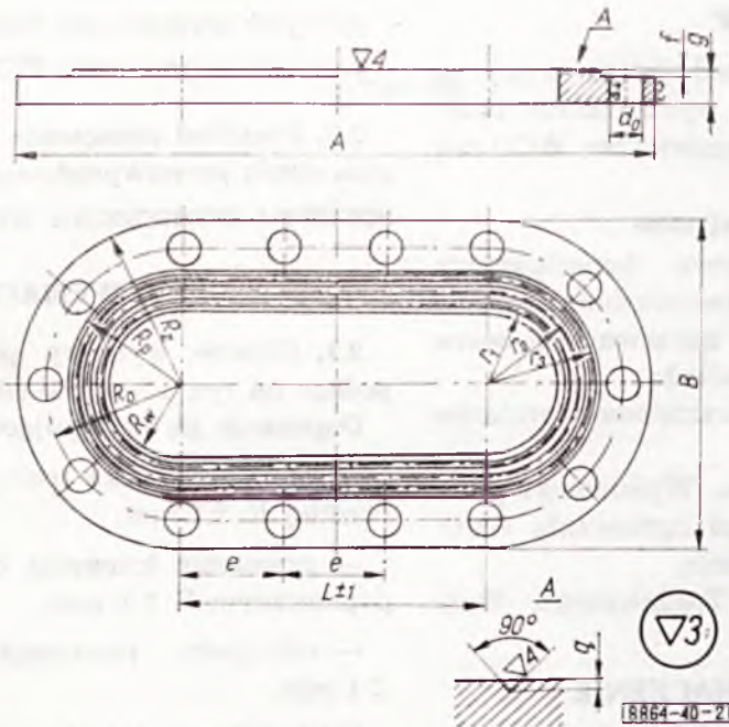
Rys. 2. Koinierz owalny pokrywy wymiennika WCO
