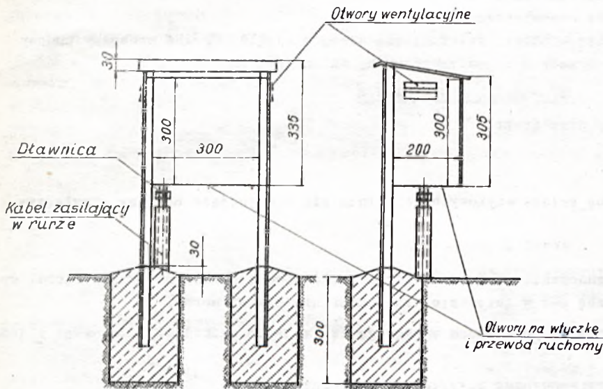
Rys. 1. Telefoniczne przyłącze wolnostojące
