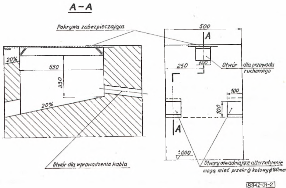
Rys. 2. Wnęka telefonicznego przyłącza nabrzeżowego
