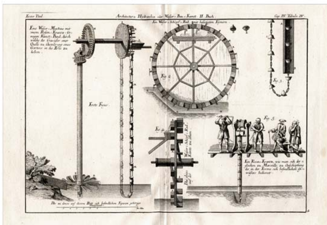
Urządzenia hydrauliczne. W: Belidor Bernard Forest de: Architectura hydraulica, oder, die Kunst das Gewässer [...] Augsburg, 1740
