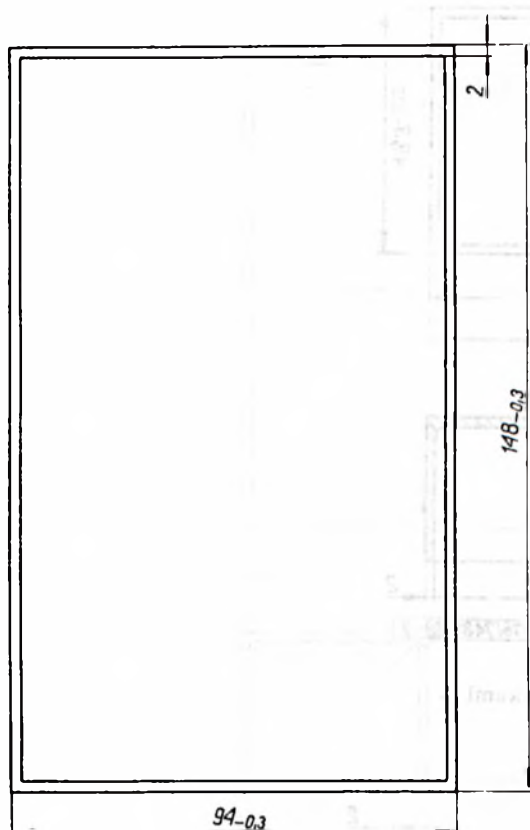
Rys. 9 Wkład jednokróbkowy 2
