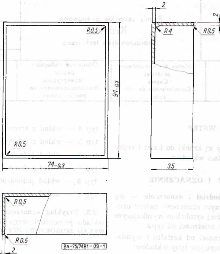
Rys. 1. Wkład jednokróbkowy
