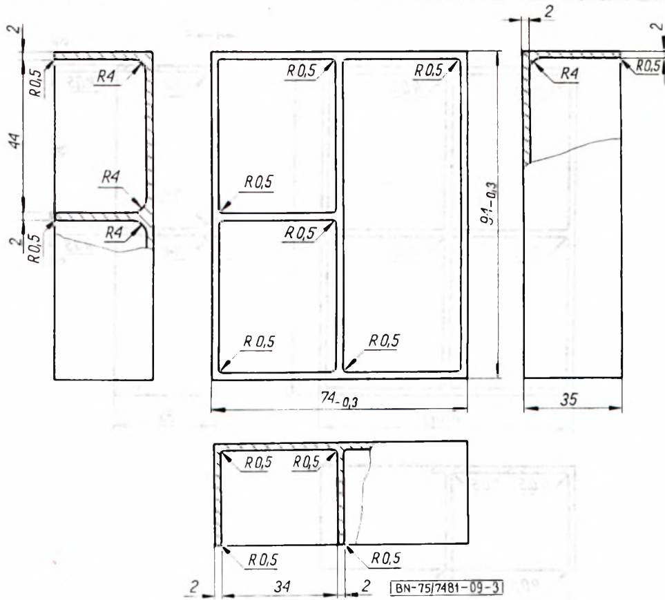
Rys. 3. Wkład z trzema króbkami A
