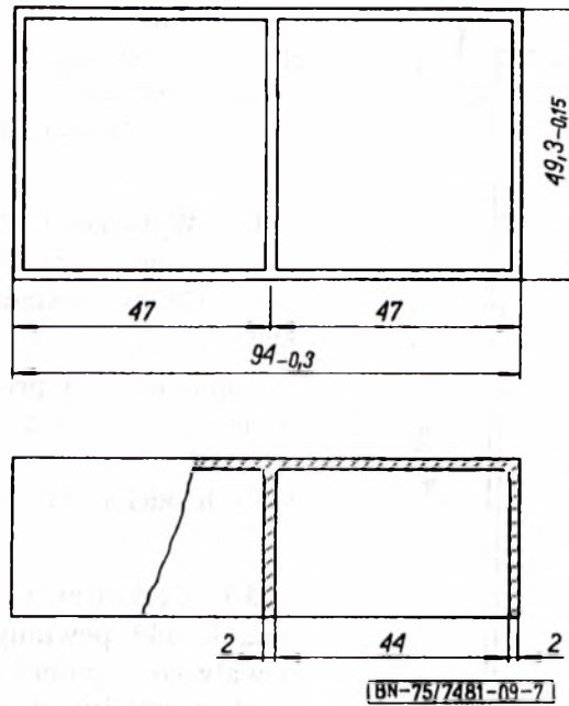
Rys. 7. Wkład z dwoma króbkami \frac{2}{3}
