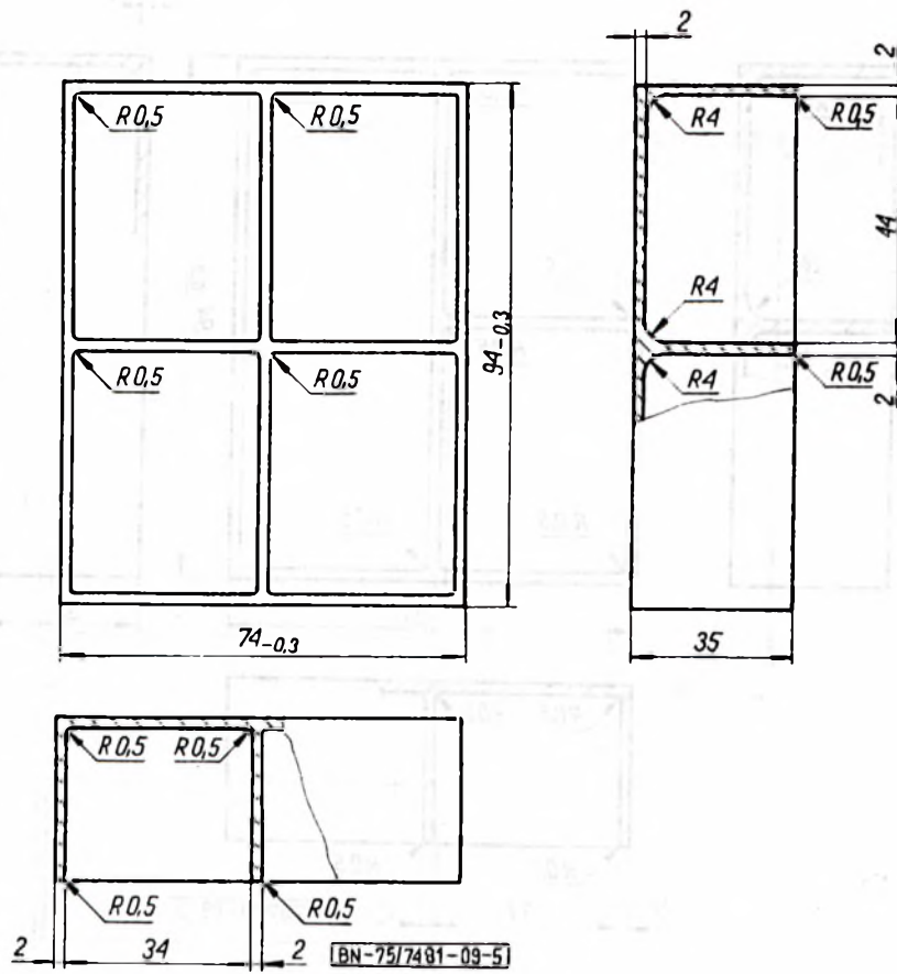
Rys. 5. Wkład z czterema króbkami
