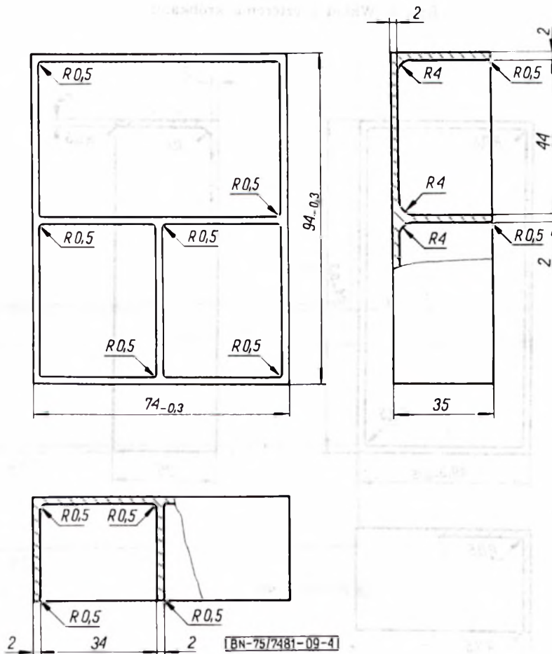
Rys. 3. Wkład z trzema króbkami A
