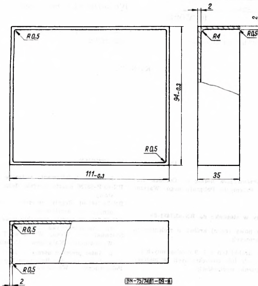
Rys. 8. Wkład jednokróbkowy \frac{3}{2}
