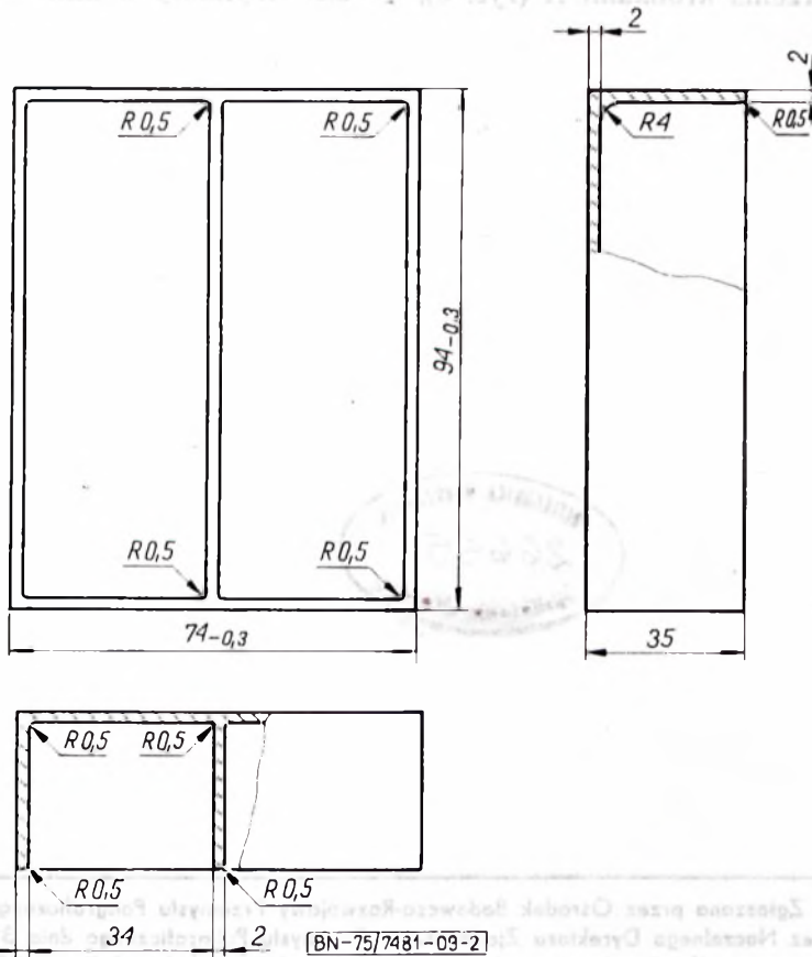
Rys. 2. Wkład z dwoma króbkami
