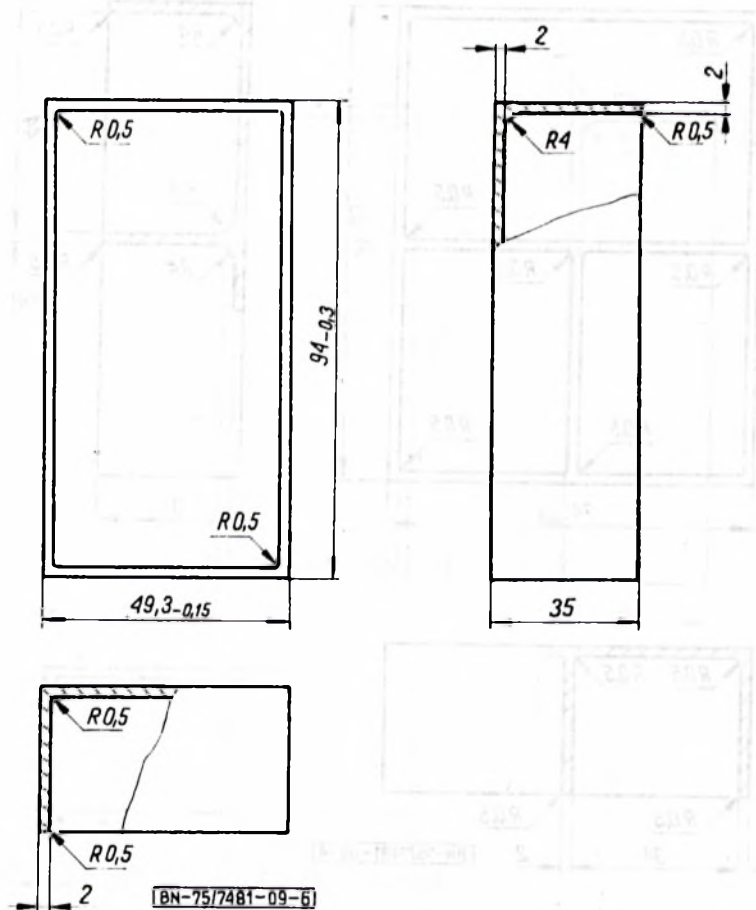
Rys. 6. Wkład jednokróbkowy \frac{2}{3}
