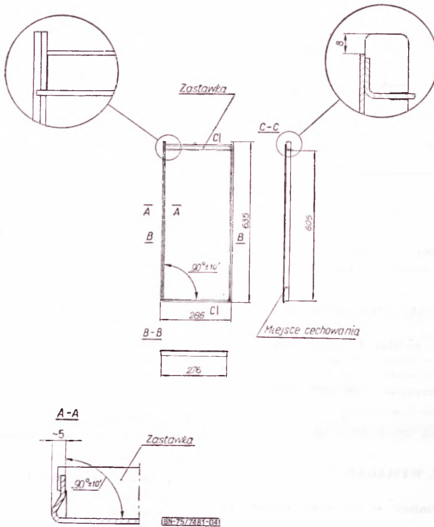
Szufelka do przechowywania składów zecerskich
