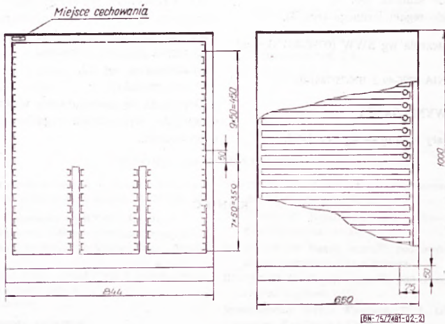
Rys. 2. Skrzynie do regału z szufladami dużymi i małymi
