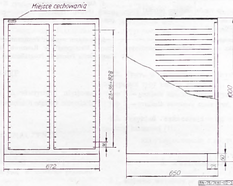
Rys. 3. Skrzynia do regału z szufelkami
