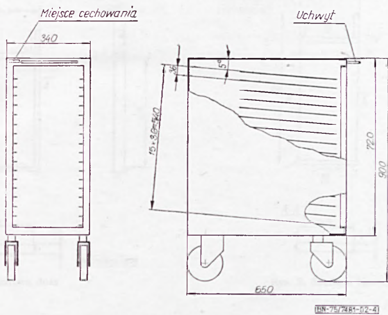
Rys. 4. Skrzynia do regału jeźdnego (wózka) z szufelkami
