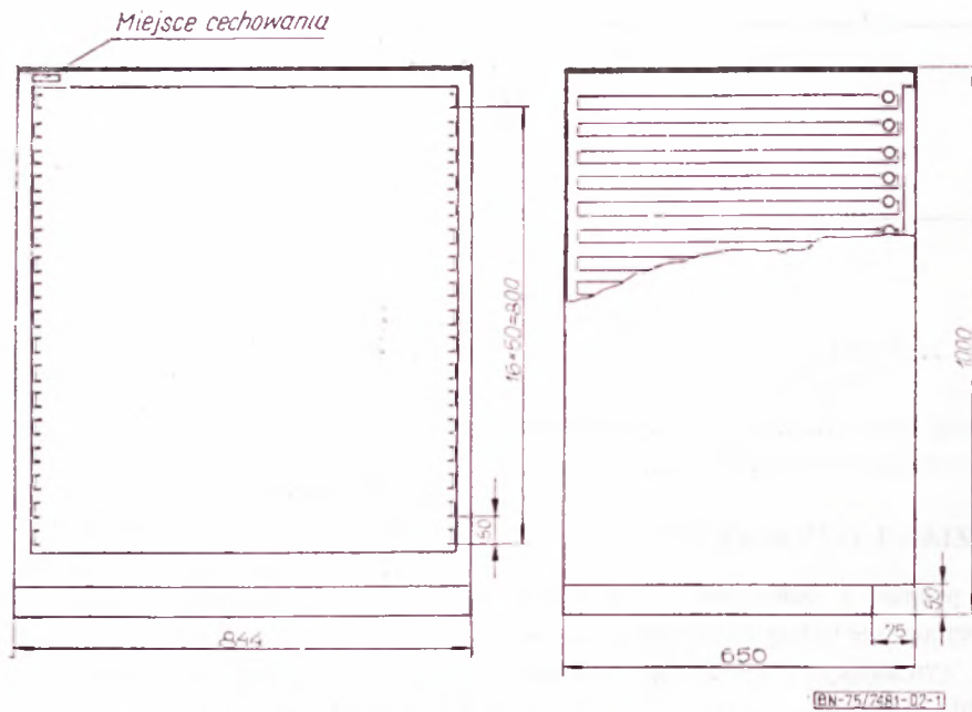
Rys. 1. Skrzynia do regałów z szufladami dużymi i do desek
